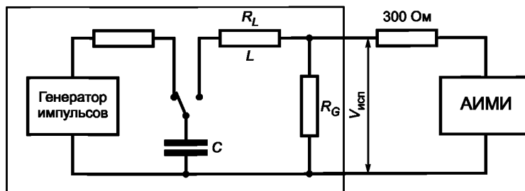
Рисунок 1 — RCL контур для оценки дефибрилляции
