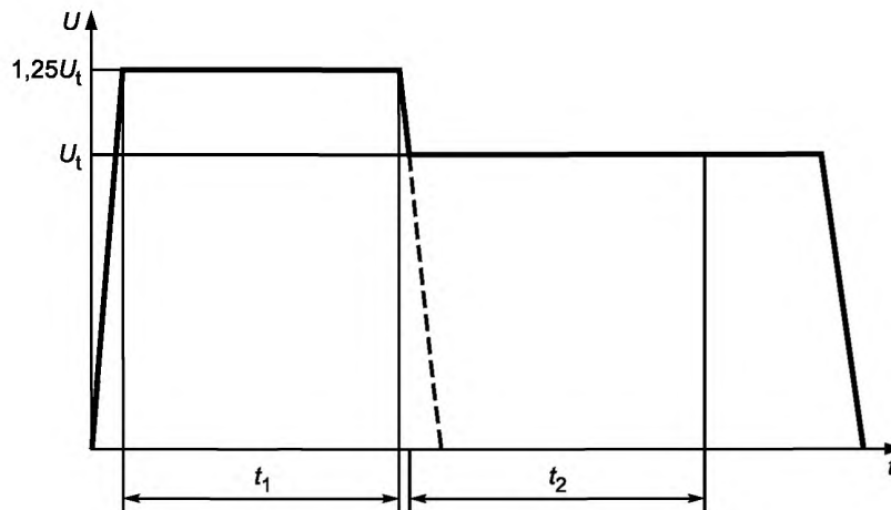
Рисунок 3 – Испытательное напряжение
