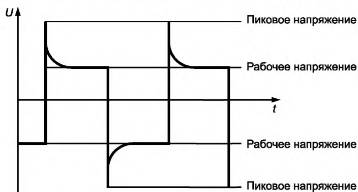
Рисунок 1 — Повторяющееся пиковое напряжение
