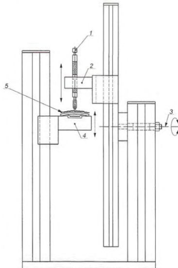
Рисунок J.2 – Пример испытательной установки
