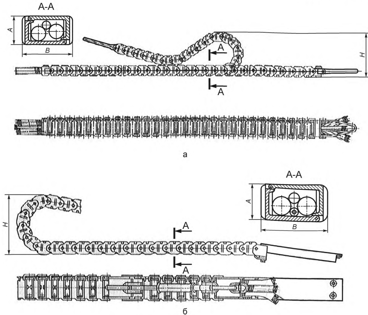
Рисунок 1 — Исполнение кабелеукладчика
