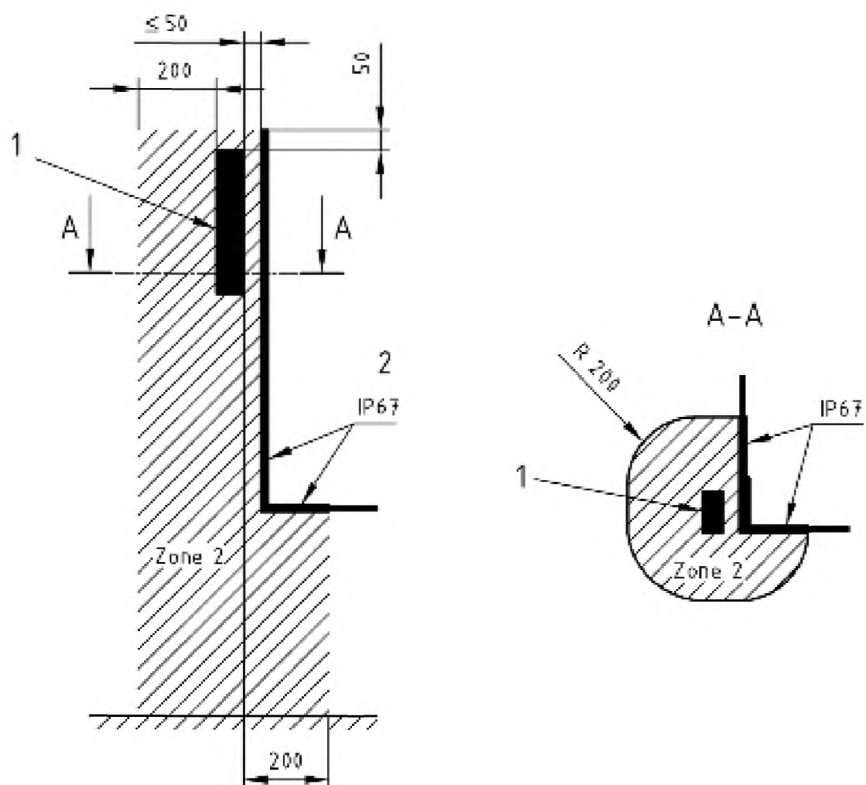
Рисунок 3 – Топливораздаточный кран снаружи кожуха на расстоянии \leq 50 мм
