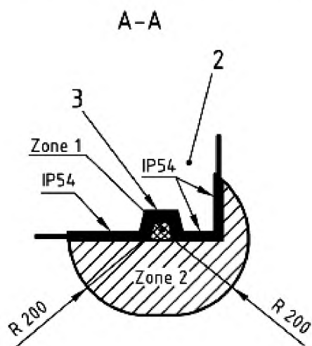
Рисунок 5 – Зона колодки топливораздаточного крана, вид сбоку
