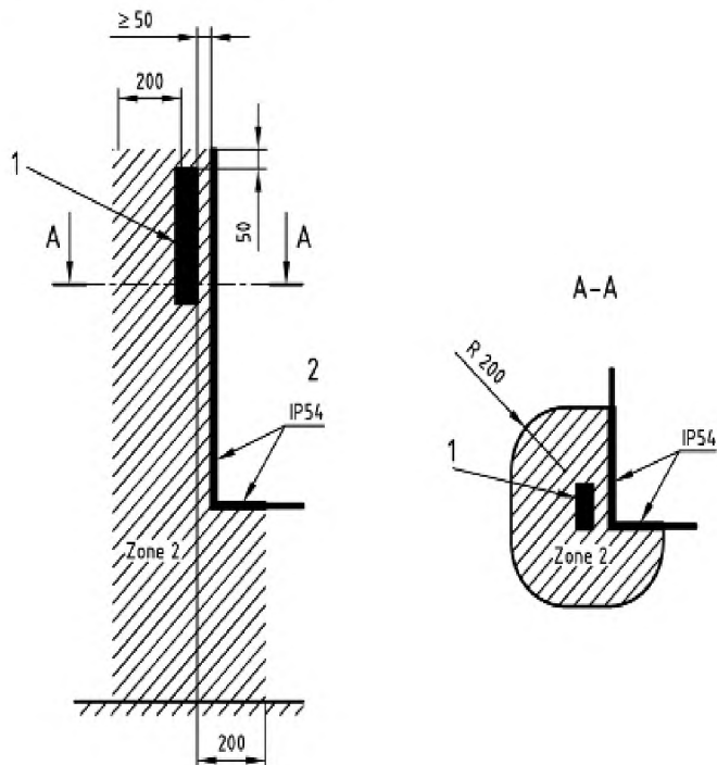
Зона 2: оборудование категории 3; 1 – топливозадаточный кран; 2 – взрывобезопасная зона
