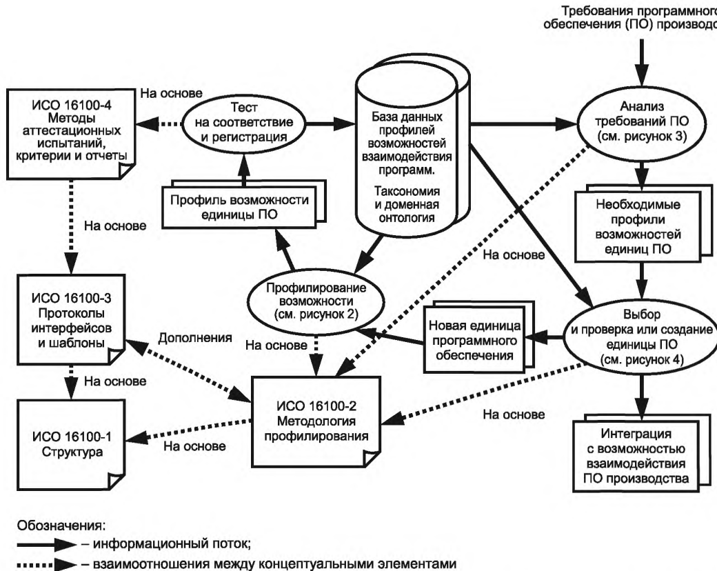
Рисунок 1 — Концепция профиля возможности интероперабельности программного обеспечения
