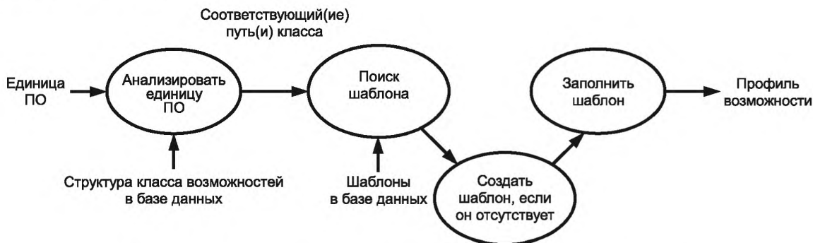
Рисунок 2 — Процесс профилирования возможности интероперабельности
