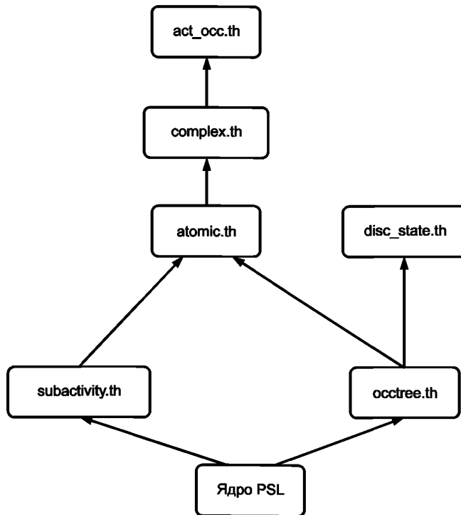
Рисунок 1 — Зависимости между наборами аксиом внешнего ядра PSL
