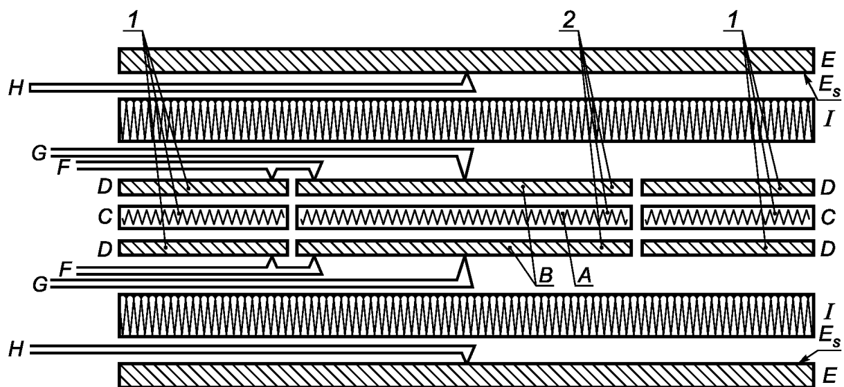
а) Прибор для одновременного испытания двух образцов
