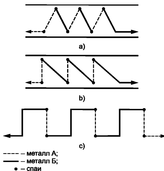
Рисунок D.7 — Примеры расположения спаев термопар термобатареи
