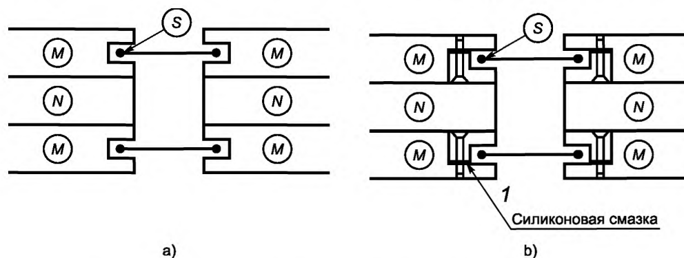
Рисунок D.2 — Расположение спейсера (прокладки) и спаев проводов уравнивающей термобатареи
