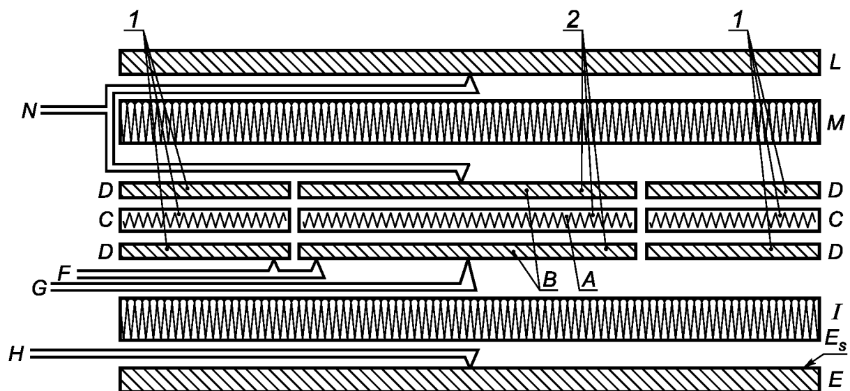
б) Прибор для испытания одного образца
