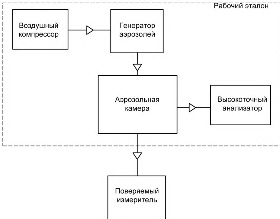
Рисунок А.1 — Схема поверки измерителей
