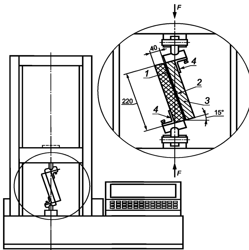
1 — образец основания; 2 — гидроизоляция; 3 — слой асфальтобетона; 4 — регулируемые опоры; F — усилие, прикладываемое к образцу
