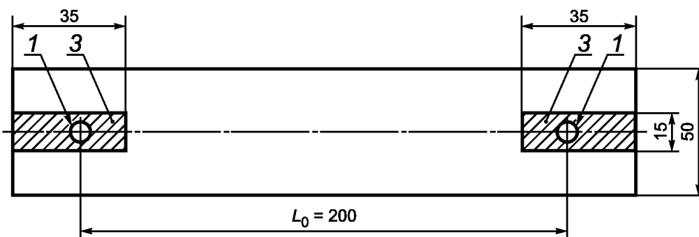
б) Образец
