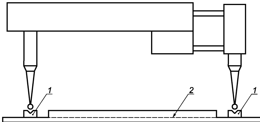
а) Экстензометр
