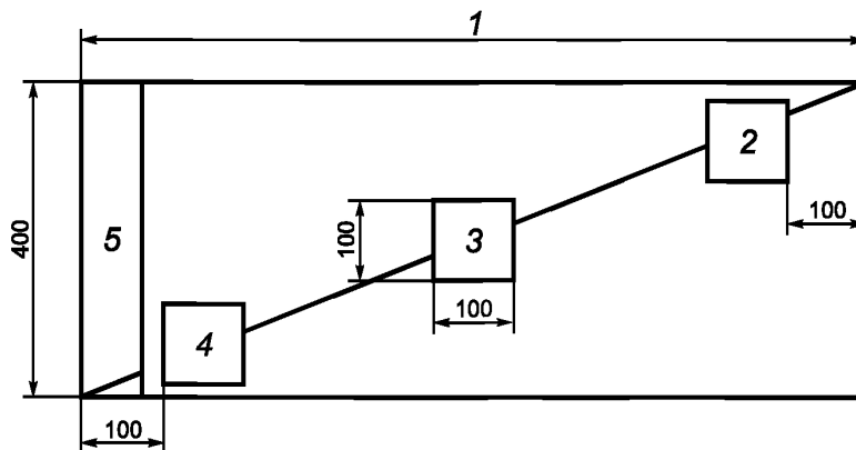
1 — ширина полотна материала; 2, 3, 4 — вырезаемые образцы; 5 — кромка
