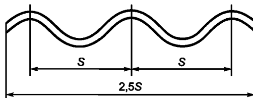
Рисунок 18 — Схема образца из волнистой части детали
