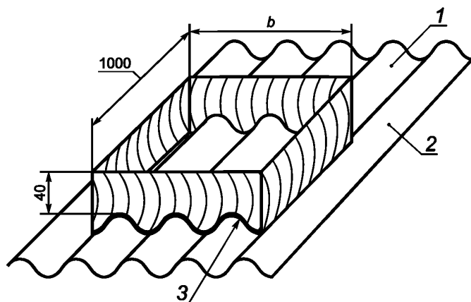
Рисунок 23 — Рама для определения водонепроницаемости
