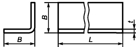
Рисунок 9 — Равнобокая угловая деталь
