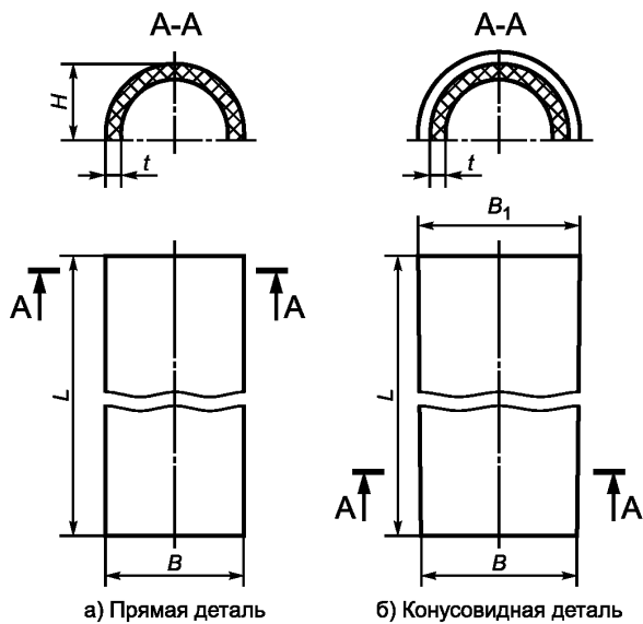
Рисунок 7 — Арочные коньковые детали
