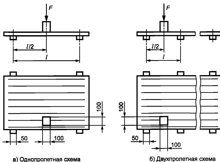
а) Однопролетная схема
