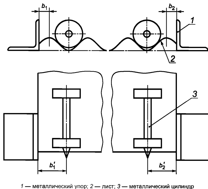
Рисунок 17 — Схема измерения ширины перекрывающей (перекрываемой) кромки
