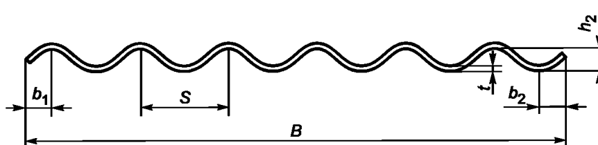
Рисунок 4 — Профиль листа 40/150 с симметричными кромками
