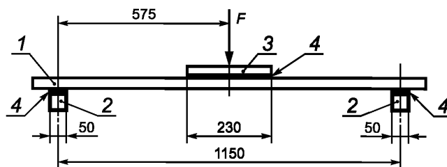
1 — лист; 2 — опора; 3 — планка; 4 — прокладка
