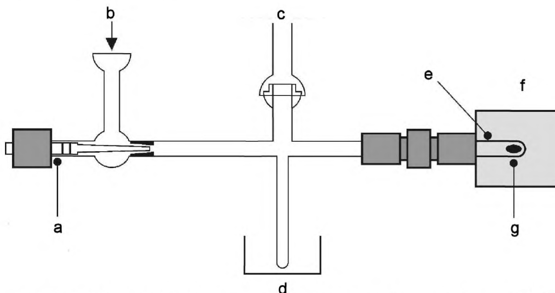
а – ампула с пробой в виде CO 2 ; б – H 2 ; в – датчик давления; г – электронный охлаждающий элемент (-18 °C для улавливания H 2 O); е – кварцевая трубка; ф – графитовая печь (600 °C); г – порошок Fe
