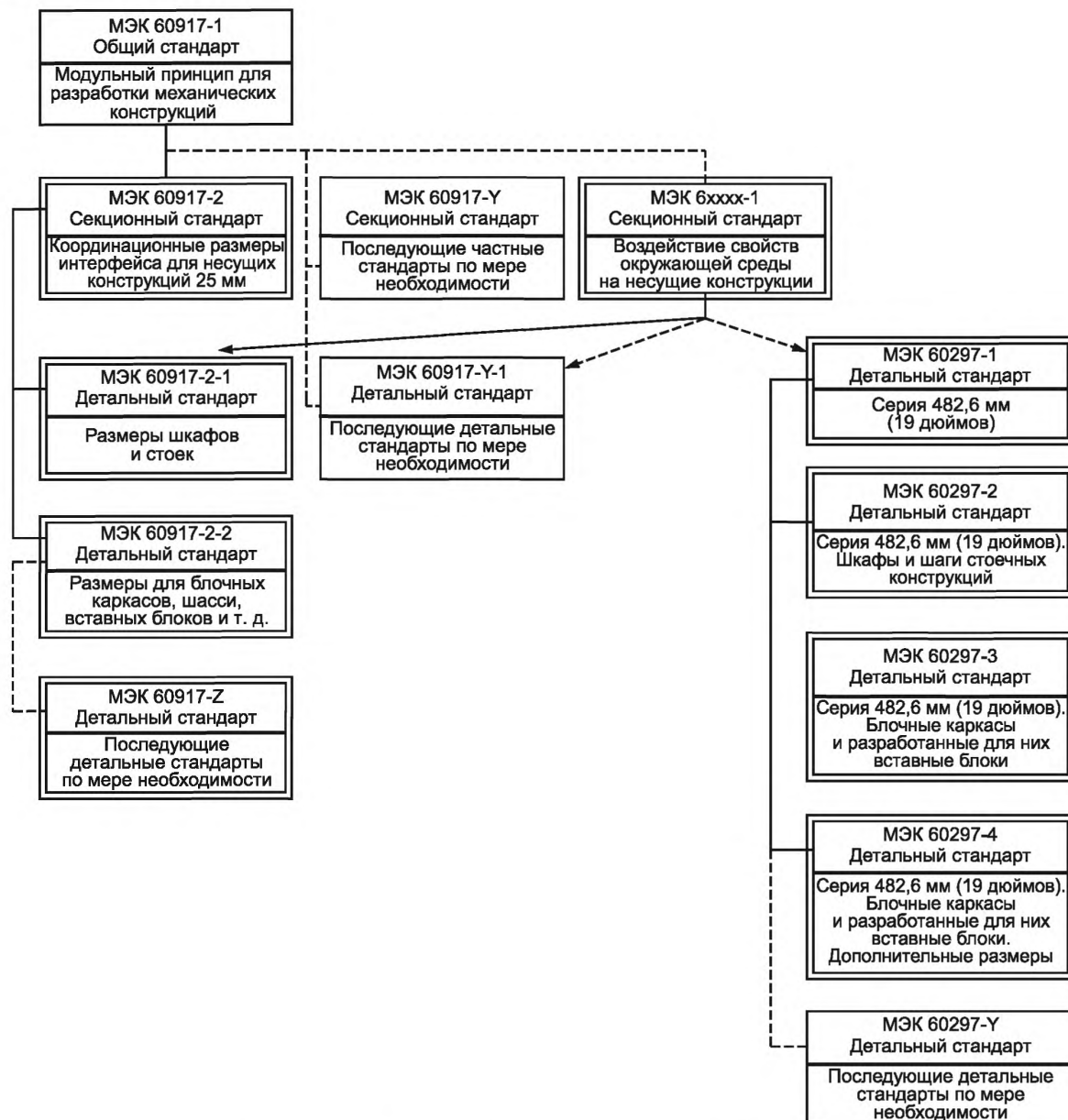
Рисунок 13 — Структура стандартов на несущие конструкции
