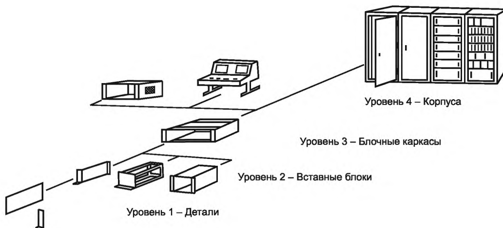
Рисунок 12 — Уровни исполнения несущих конструкций для электронного оборудования 1)
