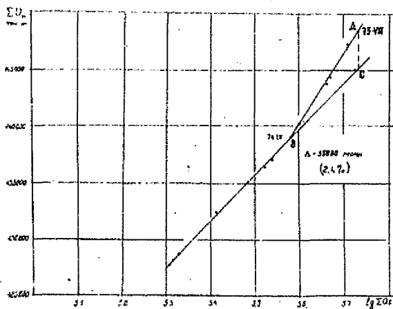
Рис. 7. Зависимость накопленного объема добытой нефти \Sigma Q_n от логарифма накопленной добычи воды \Sigma Q_b по V-VI участкам Азнакаевской площади.
