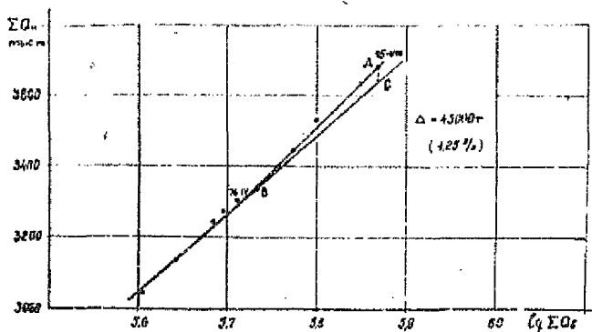
Рис. 6. Зависимость накопленного объема добытой нефти \Sigma Q_n от логарифма накопленной добычи воды \Sigma Q_b по II участку Азнакаевской площади.
