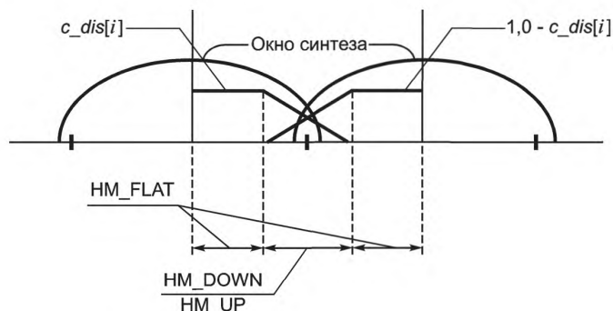
Рисунок 2 — Окно синтеза для прерывающегося шага
