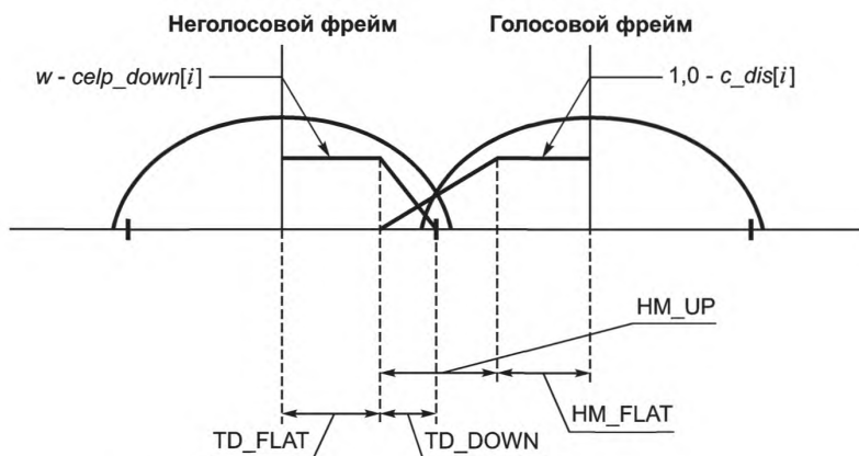
Рисунок 3 — Окно синтеза для случая неречевой/речевой
