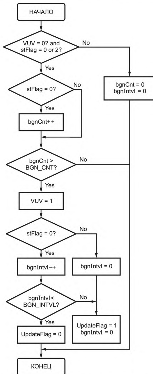
Рисунок А.1 — Блок-схема обнаружения шума
