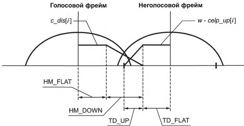
Рисунок 4 — Окно синтеза для случая речевой/неречевой
