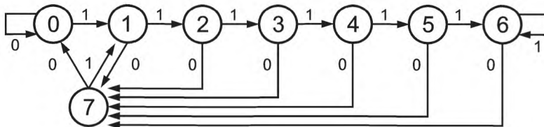
Рисунок Г.1 — Переходы состояния маскирования фрейма
