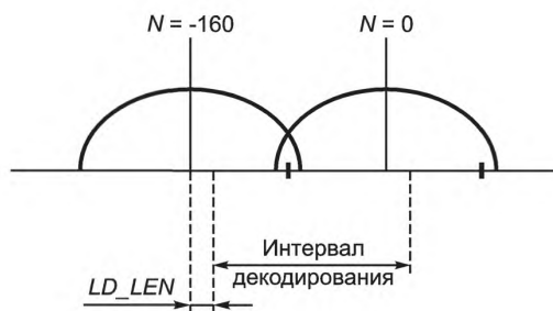
Рисунок 1 — Интервал декодирования
