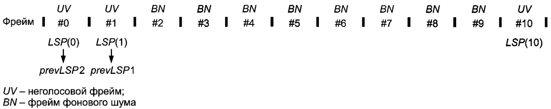
Рисунок 5 — Генерация параметров декодера для интервала фонового шума
