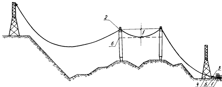
Рис. 2-6. Натягивание и визи́рование гравозащитных тросов по стреле провеса без подъема на анкерную опору
