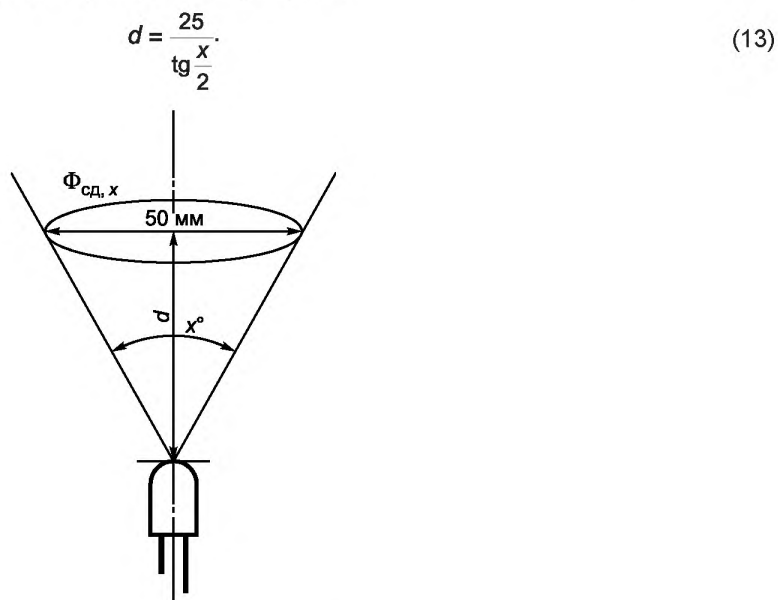
Рисунок 4 — Пояснения к определению частичного светового потока светодиодов
