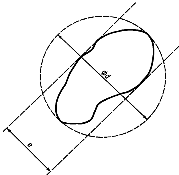
Рисунок АА.1 — Определение стандартного отверстия
