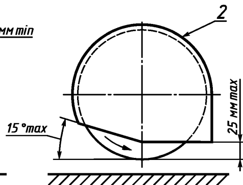
1 — испытательный стержень; 2 — минимальный контур экрана
