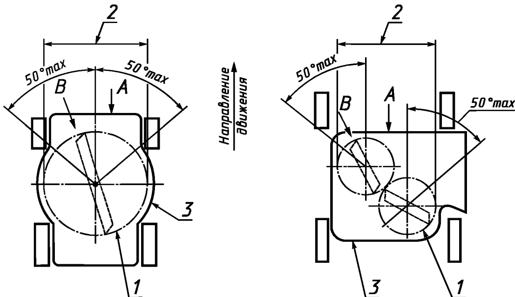
Рисунок 102 — Границы переднего отверстия одношпindelных косилок
