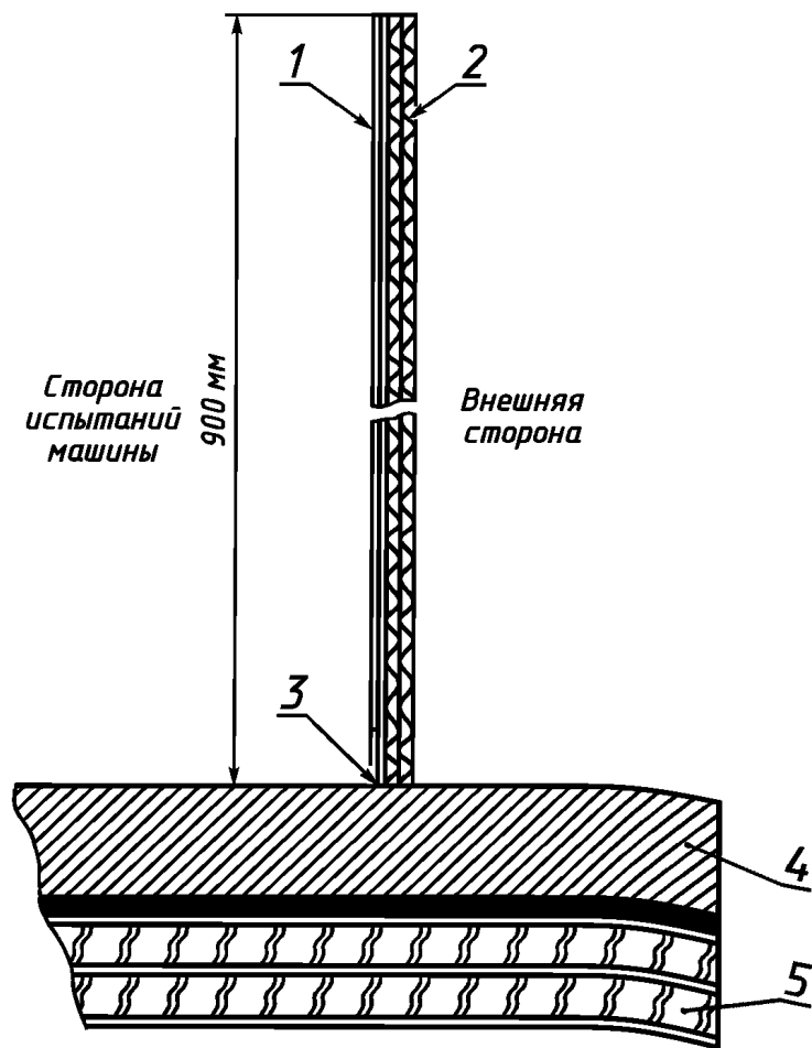
Рисунок ВВ.4 — Основание и стены испытательного ограждения
