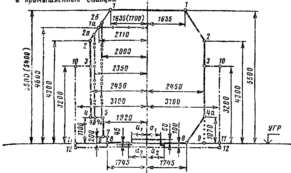
Рис. П.1.2. Габарит приближения строений Сп:
