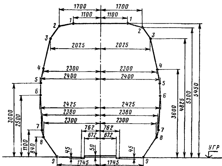
Рис. 3. Минимальное внутреннее очертание А переустраиваемых существующих инженерных сооружений (для неэлектрифицированных линий)
