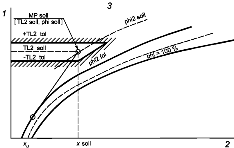
1 — массовая энтальпия воздуха h ; 2 — абсолютная влажность окружающего воздуха x\varphi ; 3 — диаграмма Мольера
