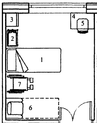
Рисунок 3 – Палата на 1 койку с местом отдыха сопровождающего
