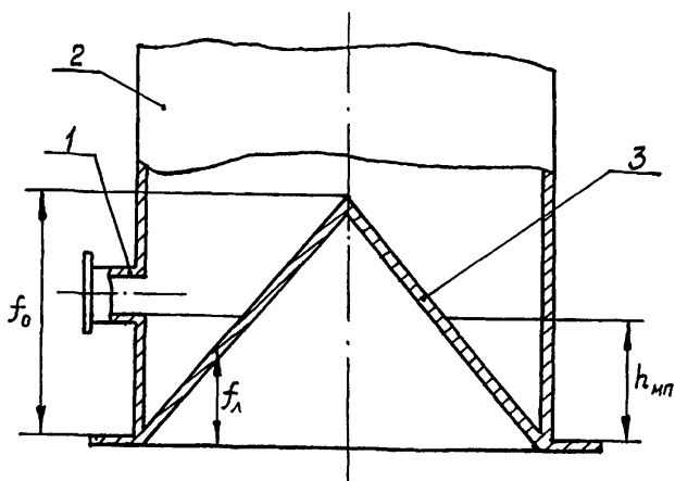
Рисунок Б.7- Схема размещения неровностей дна в пределах «мертвой» полости
