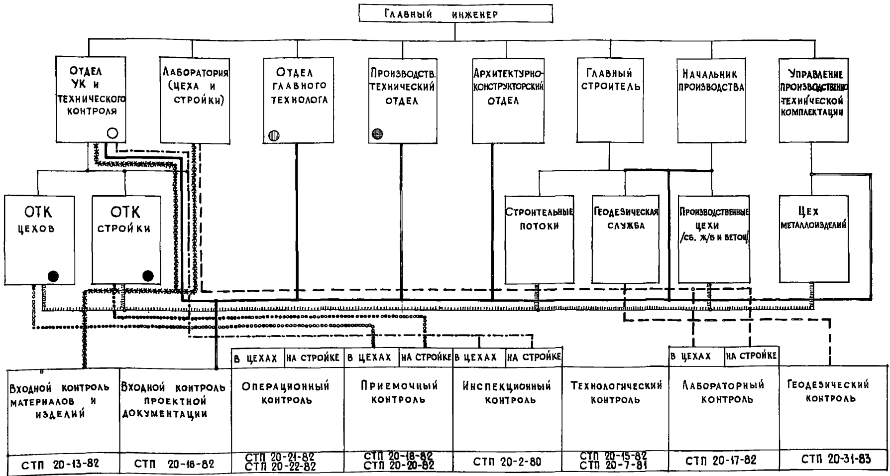
Рис. 1. Схема контроля качества на Таллинском ДСК: ○ ● ● ● — накопители информации
