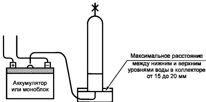
Рисунок 1 — Пример приспособления для сбора газа
