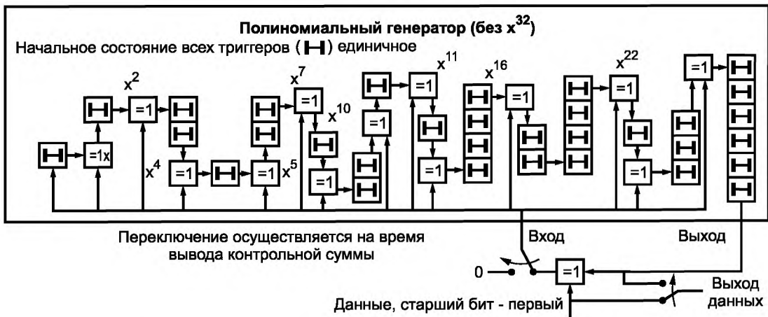
Рисунок 17 — Вычисление контрольной суммы в формирователе ТВП (PAT)
