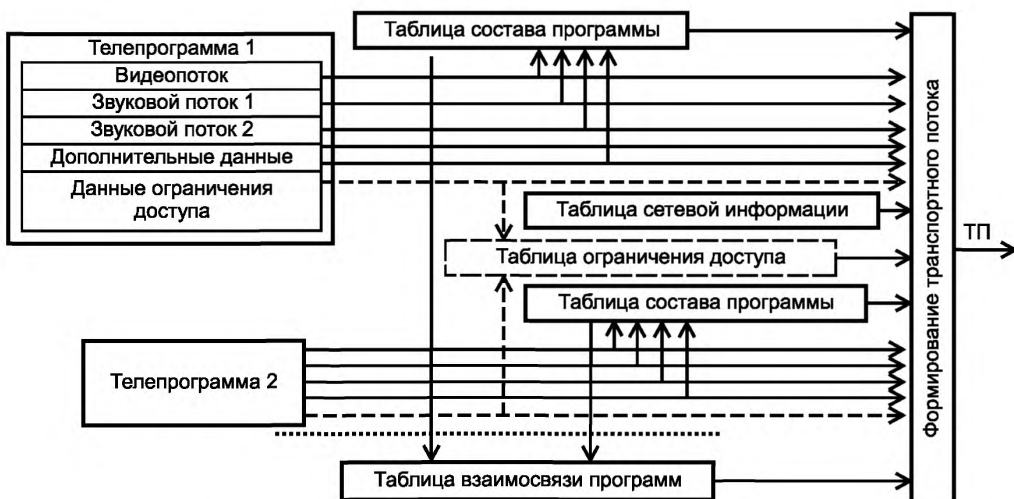
Рисунок 13 — Взаимосвязь элементов ПЗИ и телепрограмм
