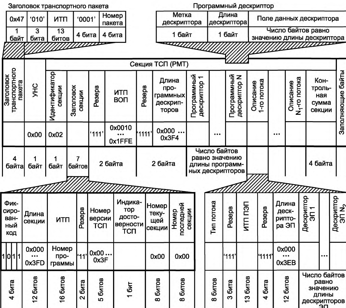
Рисунок 19 — Транспортный пакет с секцией ТСП (PMT)
