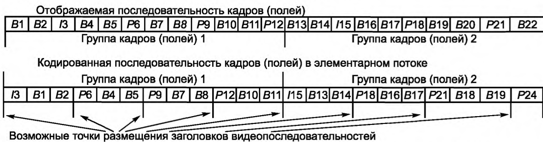
Рисунок А.16 — Отображаемая и кодированная последовательность кадров
