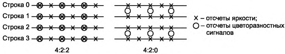
Рисунок А.2 — Форматы субдискретизации цвета 4:2:2 и 4:2:0
