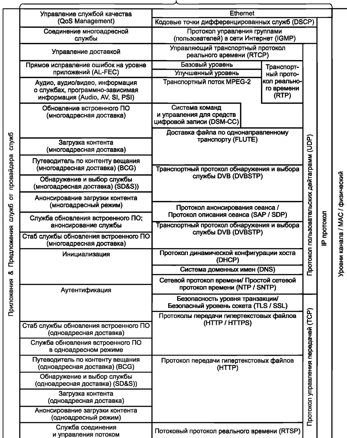
Рисунок 3 — Диаграмма стека протоколов служб DVB-IPTV
