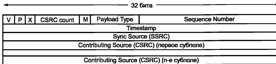
Рисунок 11 — Формат заголовка протокола RTP
