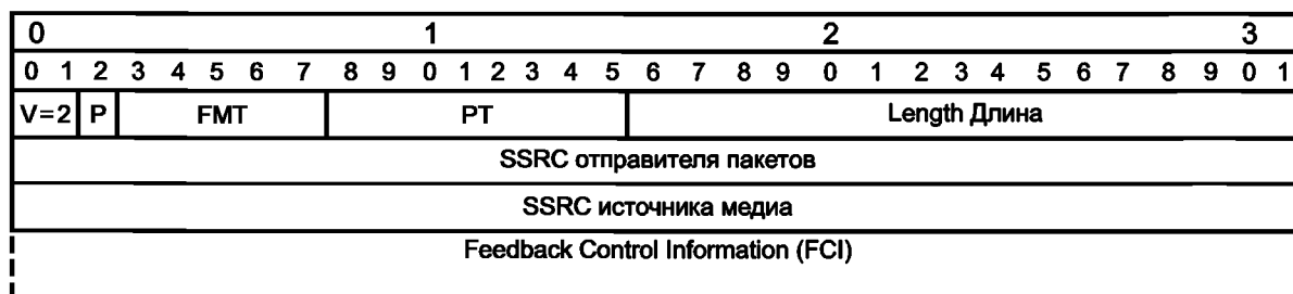
Рисунок В.4 — Формат пакета сообщения FB RTCP
