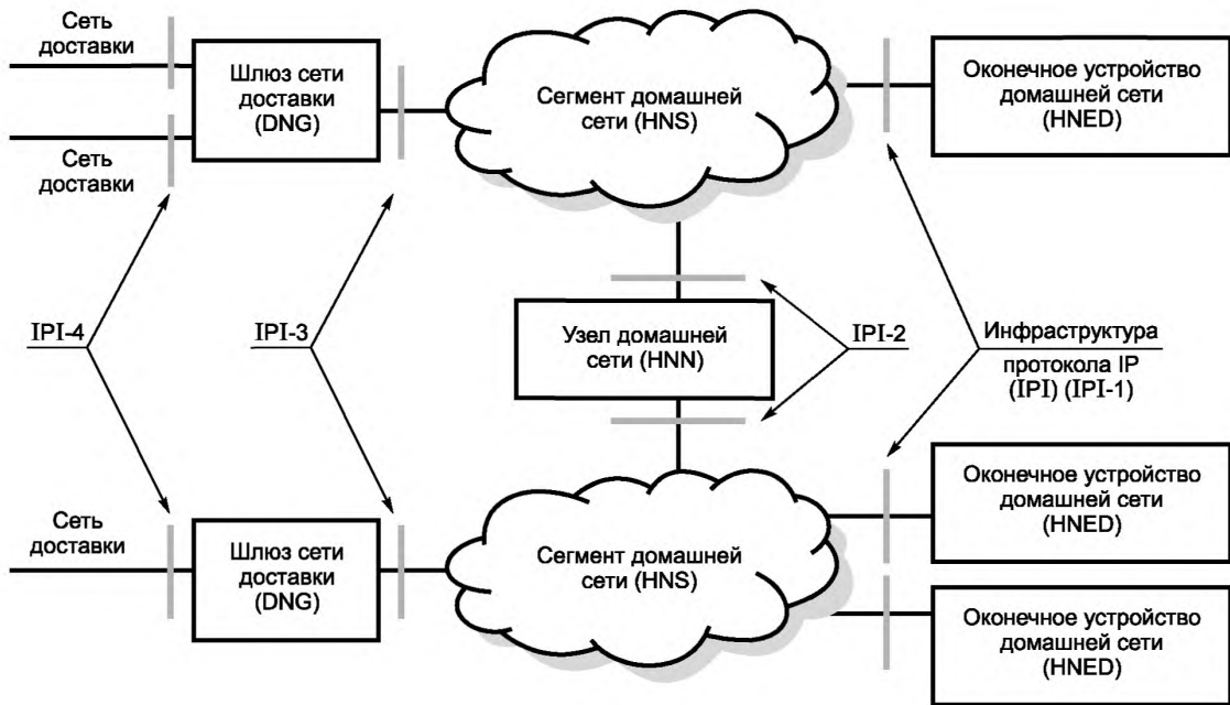
Рисунок 2 — Эталонная модель домашней сети
