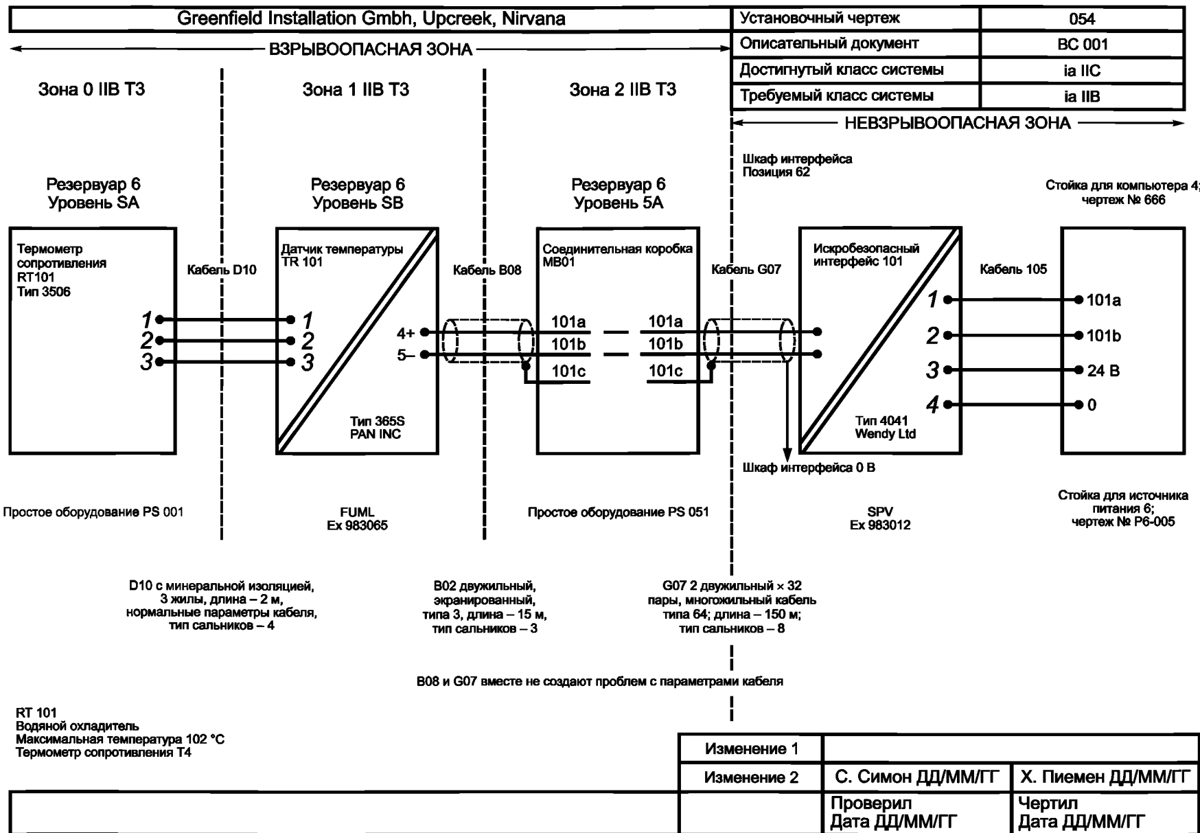
Рисунок Е.2 — Типовая схема соединений искробезопасной системы
