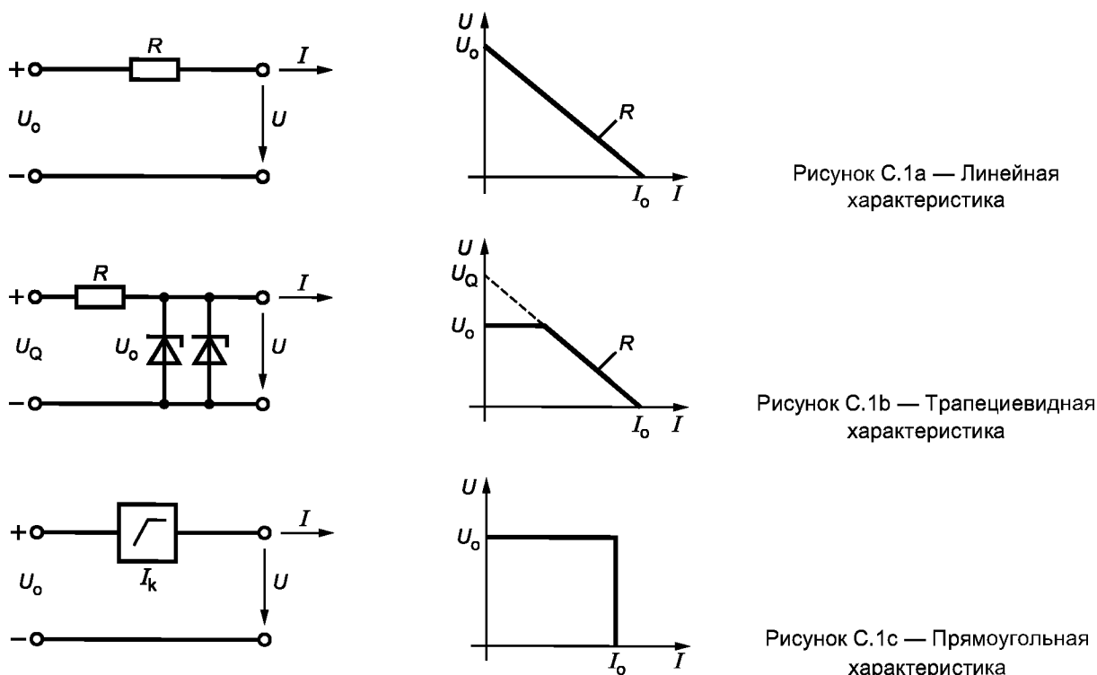
Рисунок С.1 — Характеристики эквивалентных цепей и выходов резистивных цепей
