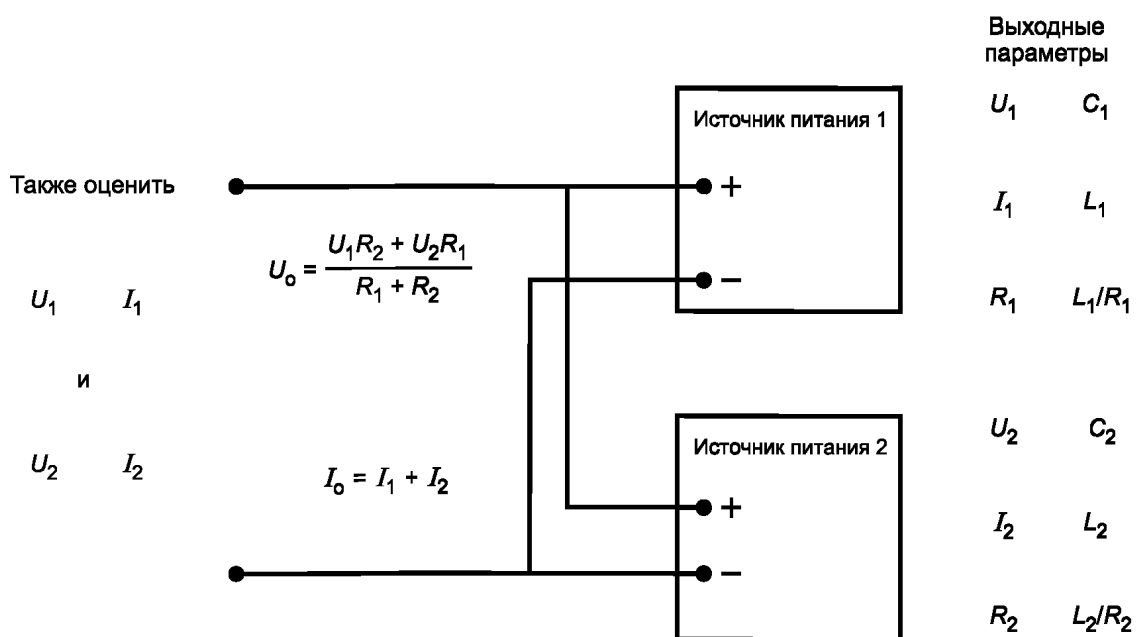
Рисунок В.2 — Источники питания, подключенные параллельно
