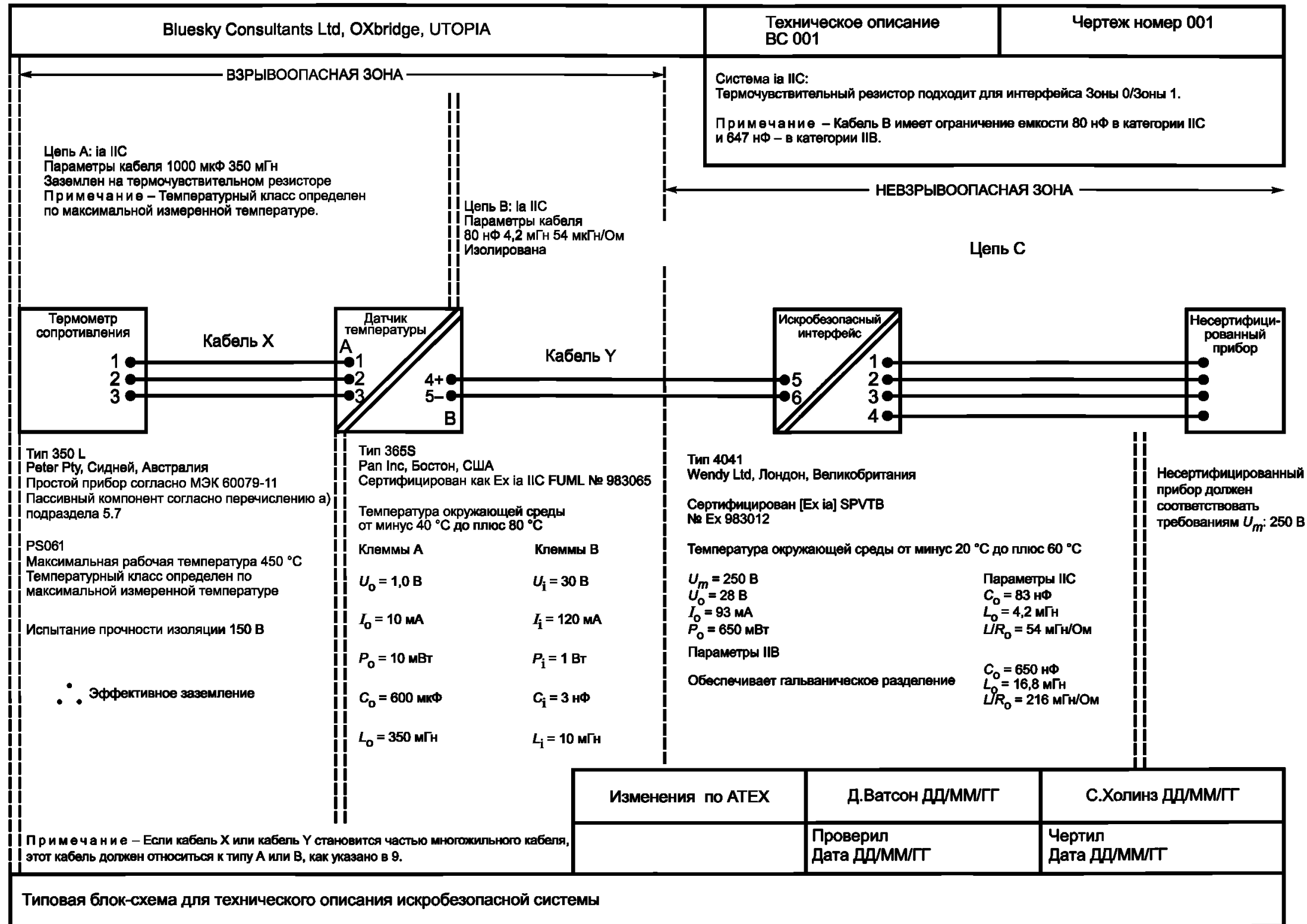
Рисунок Е.1 — Типовая блок-схема технического описания искробезопасной системы
