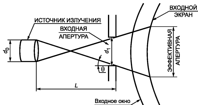
Рисунок 1 — Схема расположения ИСТОЧНИКА ИЗЛУЧЕНИЯ и ВХОДНОЙ АПЕРТУРЫ
