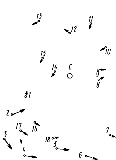
Рис. 10. Изменение цветностей при освещении люминесцентной лампой ЛД
