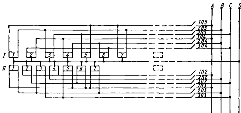
Рис. 2. Распределение нагрузки по фазам в сдвоенных рядах светильников
