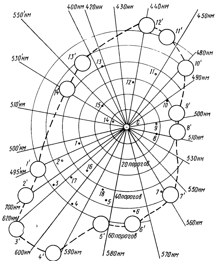
Рис. 8. Равноконтрастная диаграмма цветности v_k v_{\lambda} v_c .
