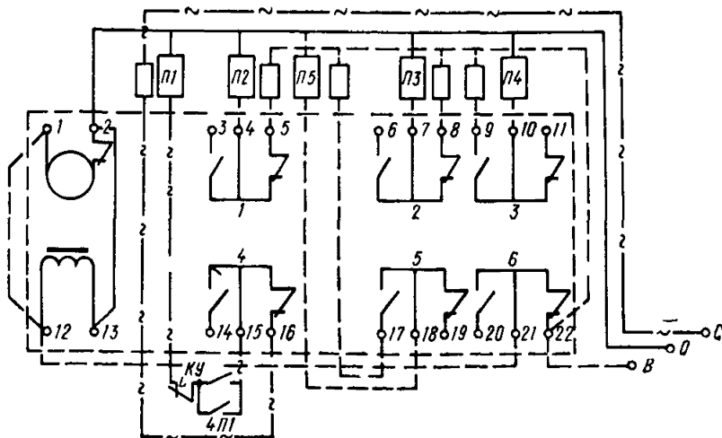
Рис. 3. Принципиальная схема подключения реле времени ВС-10-67
