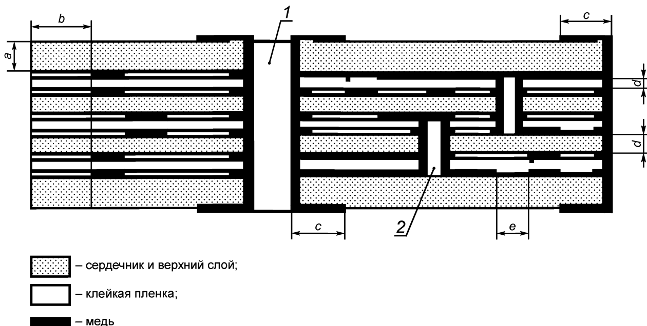
1 — сквозной контакт для заделки; 2 — сквозной контакт для соединения печатных проводников к слоям
