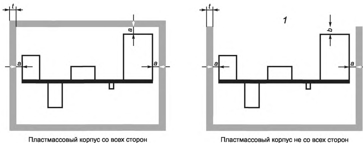
Рисунок 3 — Расстояния между стенкой или наружной поверхностью компаунда и элементами или проводниками
