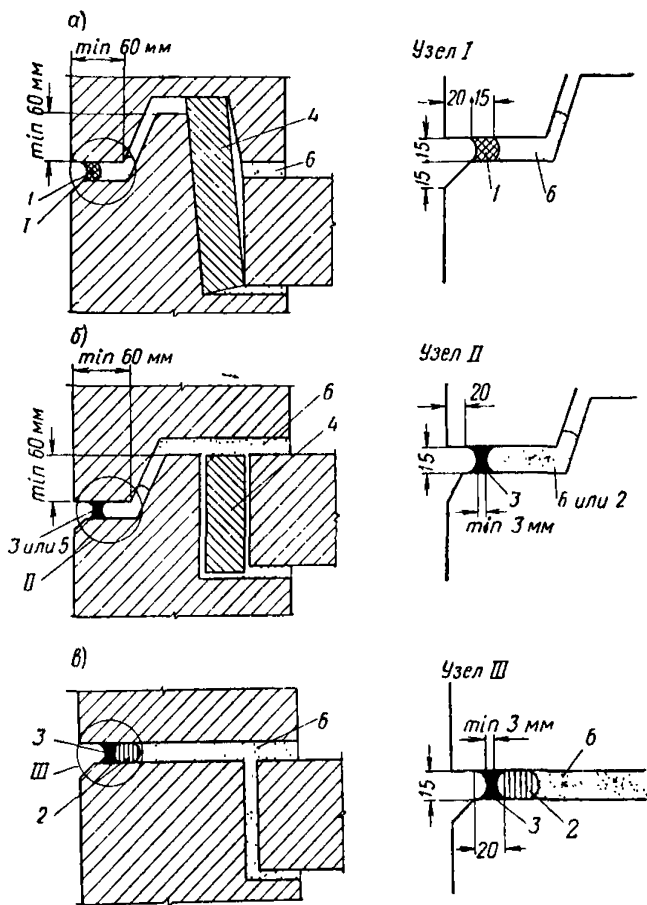
Рис. 4. Примеры герметизации и утепления горизонтальных стыков
