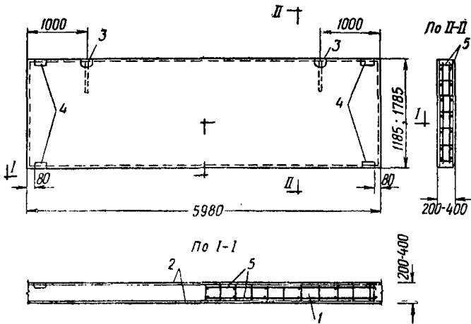
Рис. 10. Пример конструкции однослойной панели при ленточной разрезке
