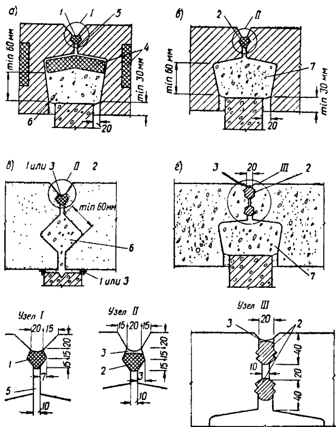
Рис. 5. Примеры герметизации и утепления вертикальных стыков
