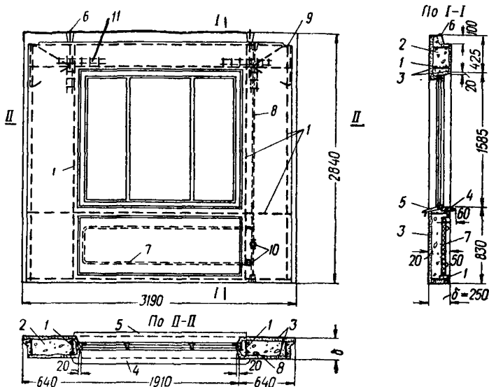
Рис. 1. Пример конструкции однослойной панели
