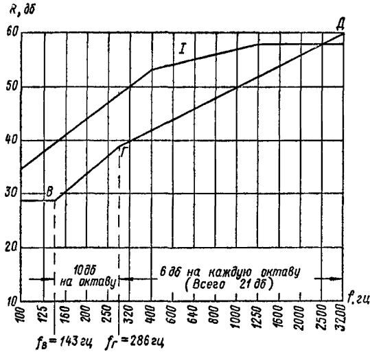
Рис. 96. Построение частотной характеристики звукоизолирующей способности шлакобетонной стены
