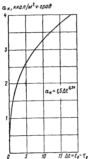
Рис. 51. Кривая для определения коэффициента теплоотдачи конвекцией теплообмена конвекцией теплообмена конвекцией стены
