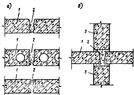
Рис. 76. Схемы сопряжений панелей перекрытий
