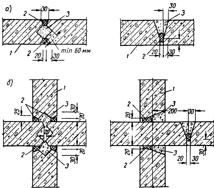
Рис. 8. Примеры решения вертикальных стыков панелей внутренних стен
