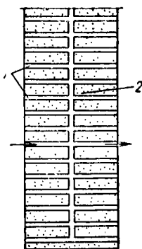
Рис. 26. Схемы устройства осушающих вентиляционных поперечных каналов
