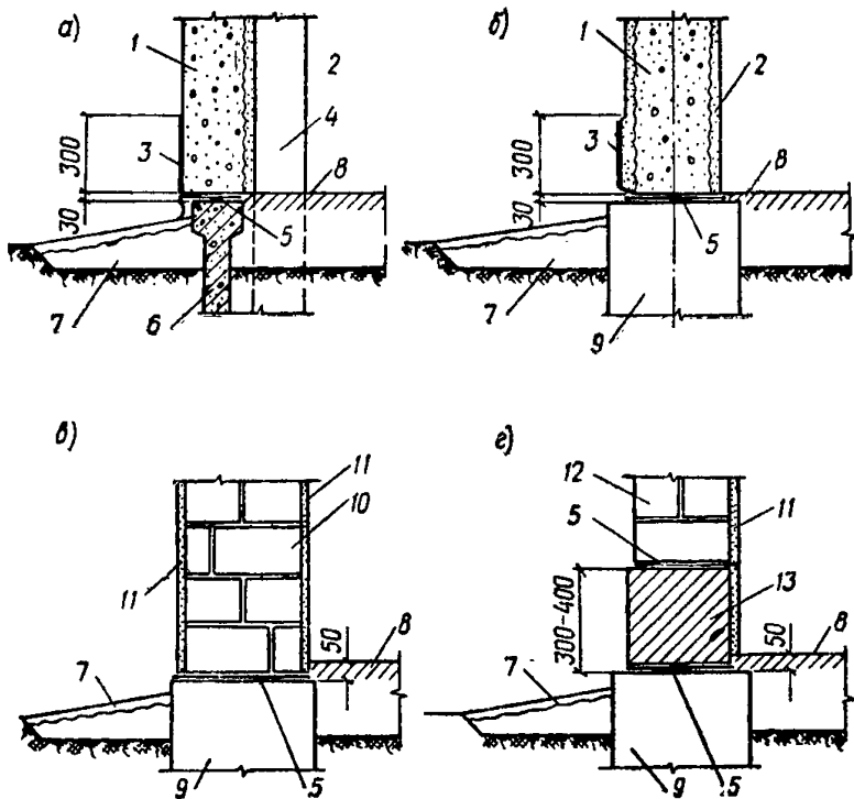
Рис. 12. Примеры гидроизоляции наружных стен сельскохозяйственных производственных зданий
