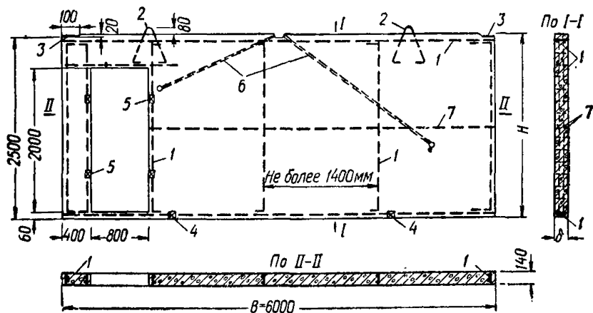
Рис. 7. Пример конструкции однослойной панели внутренней стены
