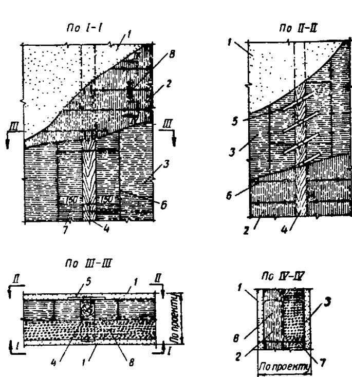
Рис. 15. Пример крепления камшитовых плит к деревянному фахверку
