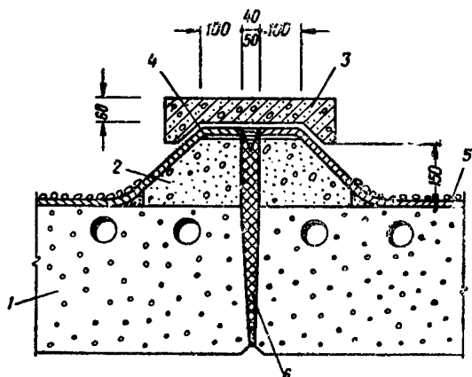
Рис. 27. Схема устройства температурно-осадочного шва
