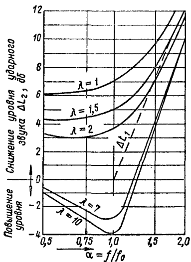
Рис. 88. График для определения \Delta L_2
