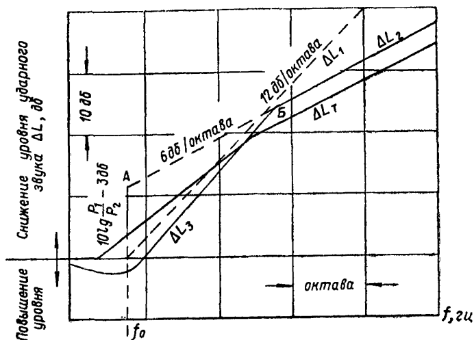
Рис. 87. Построение частотной характеристики снижения уровня ударного звука
