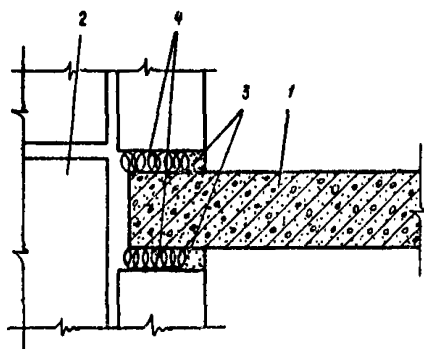
Рис. 75. Схема примыкания внутренних стен к наружным
