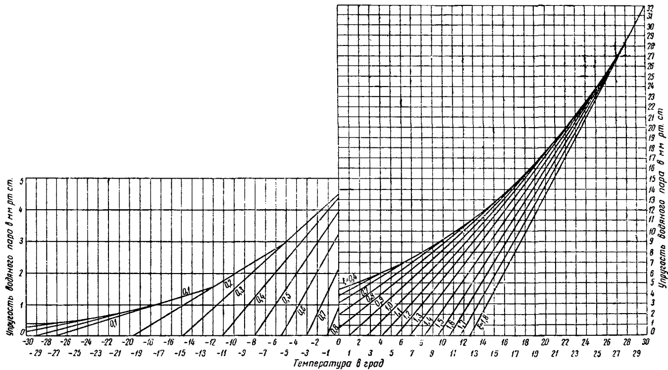
Рис. 67. График определения относительного расхода пара \xi_H
