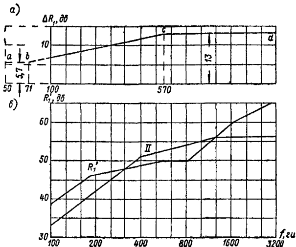
Рис. 99. Построение частотной характеристики звукоизолирующей способности раздельной стены
