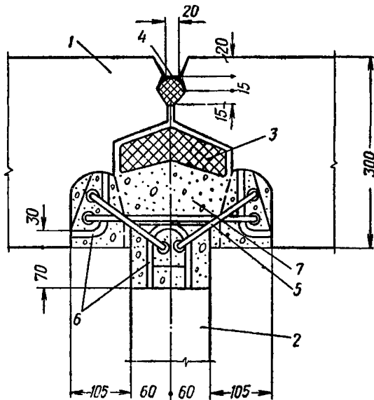
Рис. 6. Пример конструкции соединительных связей замоноличенного вертикального стыка (серии по типу проекта I-464)
