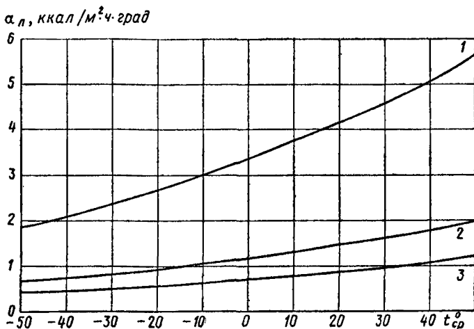
Рис. 52. Кривые для определения коэффициента теплообмена излучением \alpha_n
