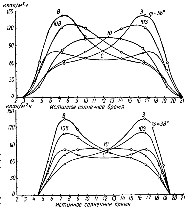
Рис. 45. Суточный ход интенсивности прямой солнечной радиации, поступающей при безоблачном небе на вертикальные поверхности различной ориентации в июне и декабре для широт 38 и 56°.
