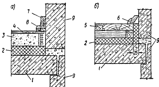
Рис. 23. Детали примыкания пола к стенам
