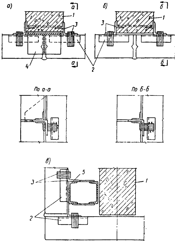
Рис. 11. Примеры крепления стеновых панелей к несущему каркасу
