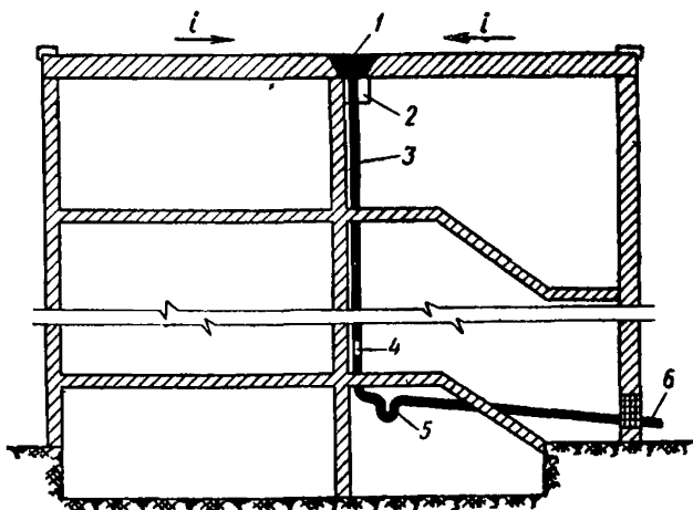
Рис. 33. Схема внутреннего водостока с наружным выпуском воды
