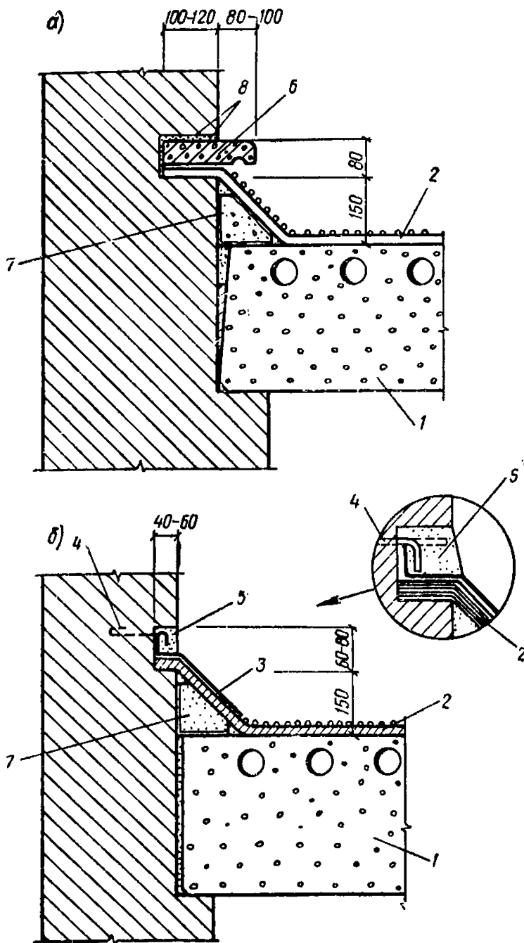
Рис. 29. Примыкания гидроизоляционного ковра к вертикальным стенам
