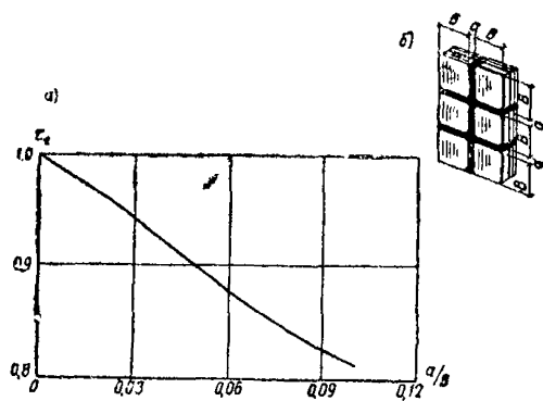
Рис. 39. График для определения коэффициента \tau_2 стекложелезобетонных ограждений
