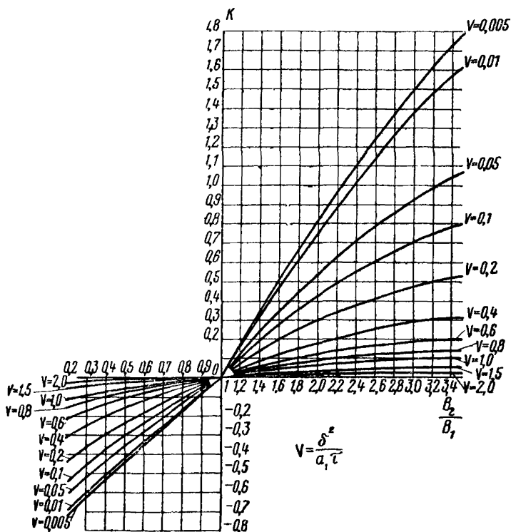
Рис. 62. Номограмма для определения безразмерного параметра K
