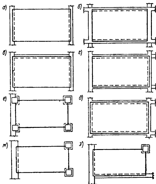
Рис. 21. Схемы опирания панелей перекрытий
