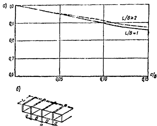
Рис. 38. График для определения коэффициента \tau_2
