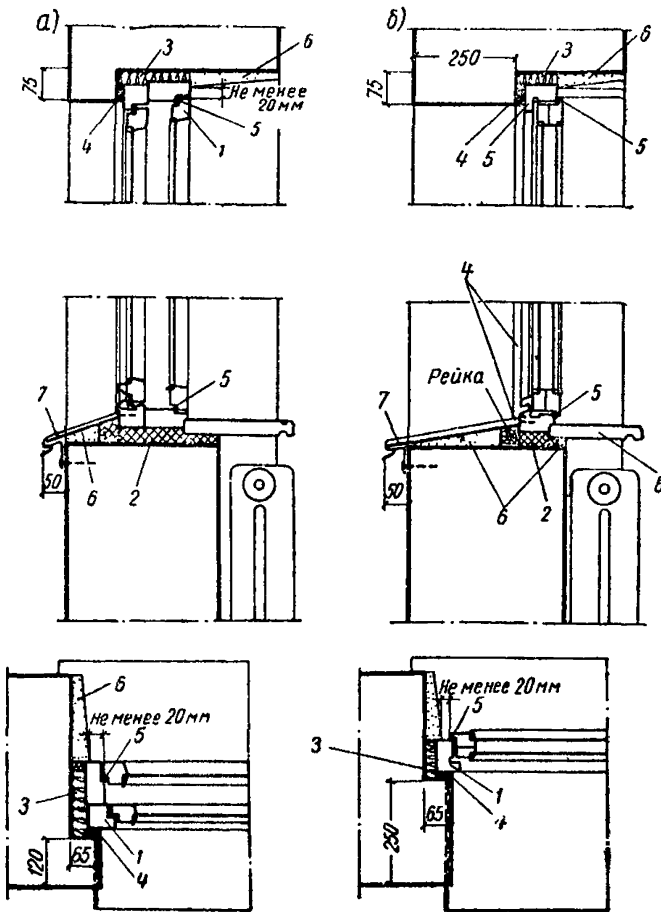
Рис. 40. Примеры установки оконных блоков в кирпичных стенах
