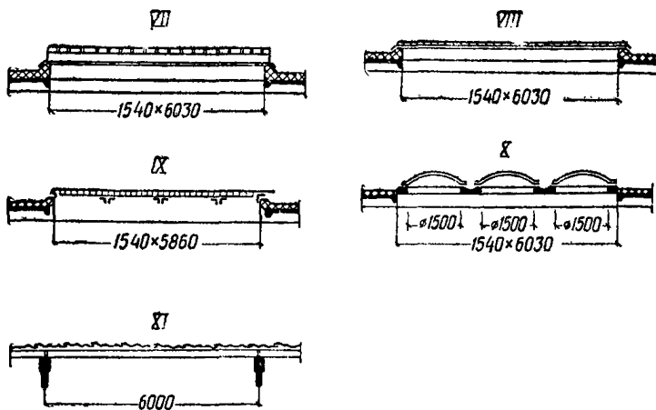
Рис. 44. Схемы зенитных фонарей с применением стеклопластиков, рекомендуемых для внедрения в промышленное строительство
