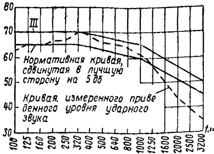
Рис. 95. Частотная характеристика приведенного уровня ударного звука
