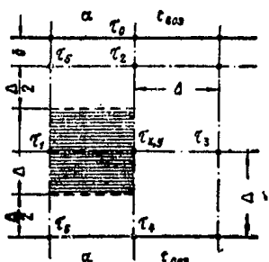
Рис. 57. К расчету температурного поля
