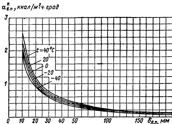
Рис. 54. Кривые для определения \alpha_{в.п}^к в горизонтальных воздушных прослойках при потоке тепла сверху вниз
