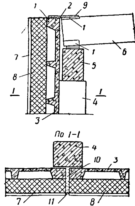
Рис. 14. Пример крепления виброкатных железобетонных панелей
