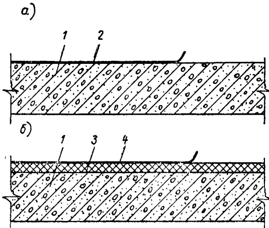
Рис. 81. Схемы полов из рулонных материалов
