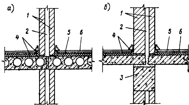
Рис. 73. Схема установки перегородок со сплошным воздушным промежутком
