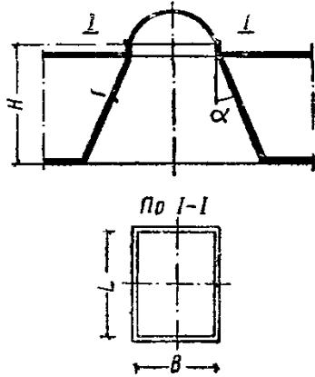
Рис. 36. Схема зенитного светопроема со светопрозрачным колпаком
