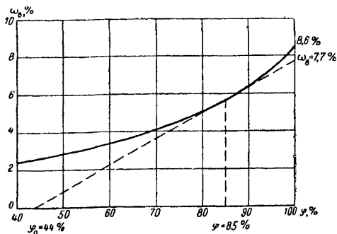
Рис. 69. Изотерма сорбции пенобетона, \gamma = 400 \text{ кг/м}^3
