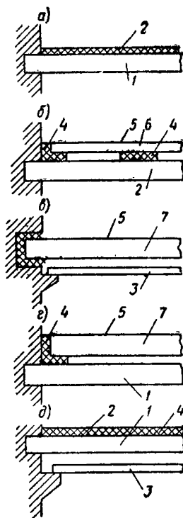
Рис. 20. Конструктивные схемы перекрытий
