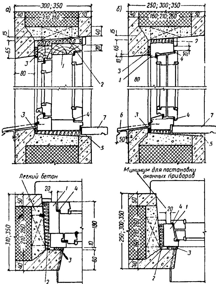
Рис. 41. Примеры установки оконных блоков в панельных стенах
