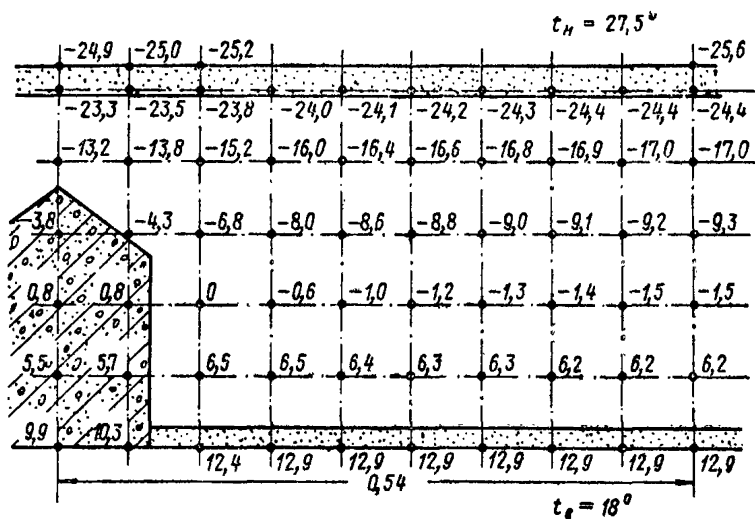
Рис. 59. Температурное поле стыка панелей
