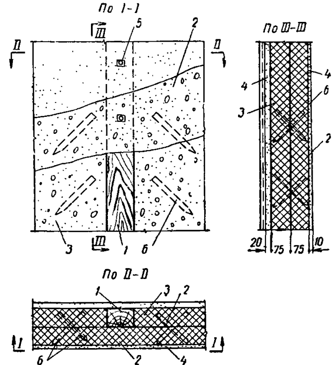
Рис. 16. Пример крепления фибролитовых плит к деревянному фахверку
