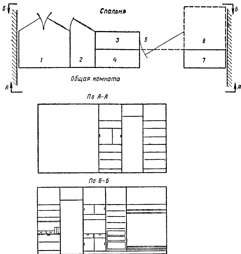
Рис. 18. Пример схемы компоновки шкафа-перегородки
