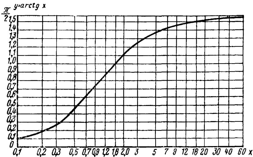
Рис. 61. Значения y = \arctg x
