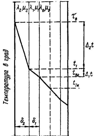
Рис. 68. Изменение температуры в многослойном ограждении
