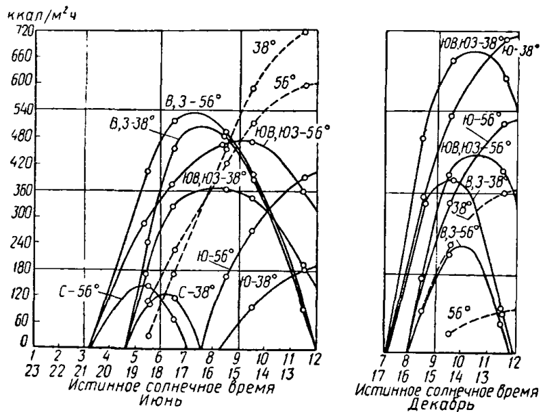
Рис. 45. Суточный ход интенсивности прямой солнечной радиации, поступающей при безоблачном небе на вертикальные поверхности различной ориентации в июне и декабре для широт 38 и 56°.
