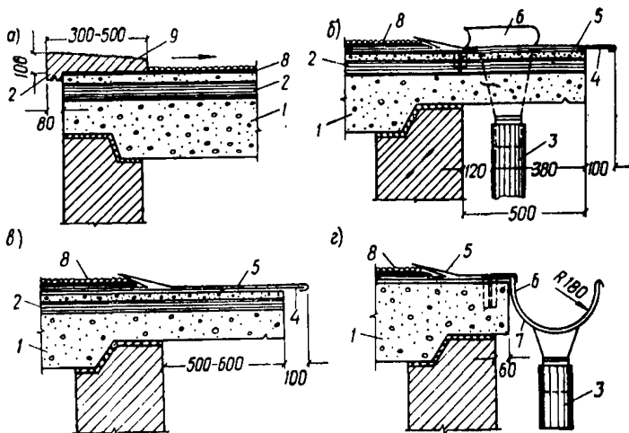
Рис. 32. Решение карнизов
