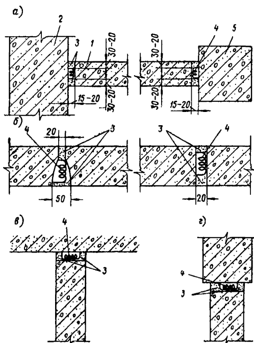
Рис. 74. Схема сопряжений перегородок с другими конструкциями
