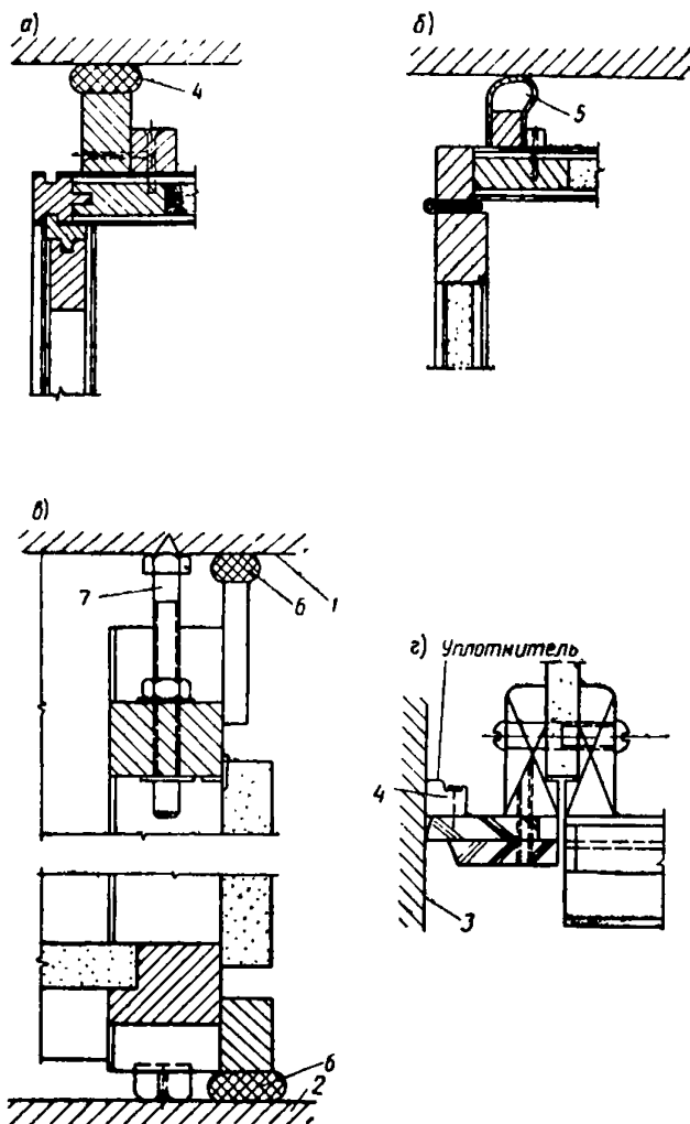
Рис. 19. Примеры решения сопряжений шкафов-перегородок с ограждающими конструкциями
