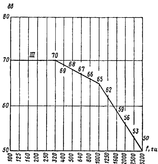
Рис. 72[2] (СНиП II-В.6-62, рис. 2). Нормативная кривая приведенного уровня ударного звука под перекрытием
