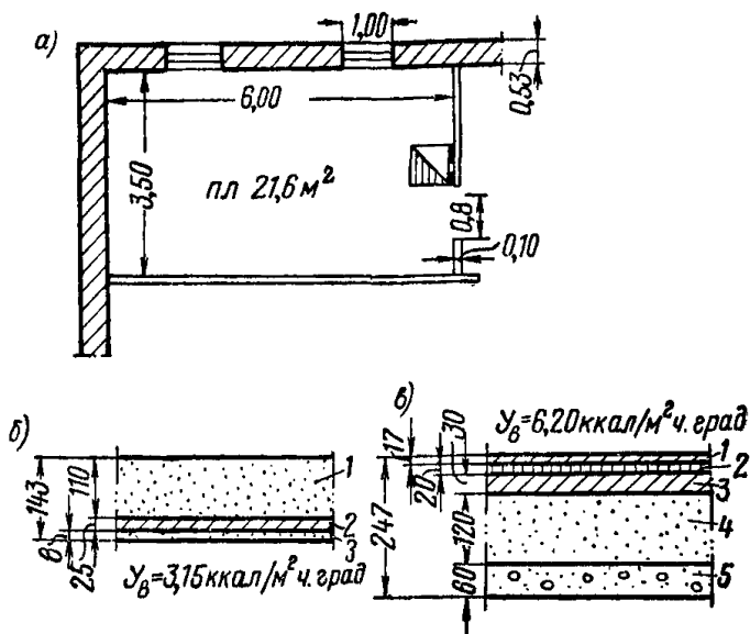
Рис. 60. План и конструкции помещения
