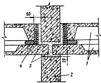
Рис. 77. Схема перекрытия раздельного типа 1 — панель перекрытия; 2 — стеновые панели; 3 — заделка раствором; 4 — полутвердая древесноволокнистая плита
