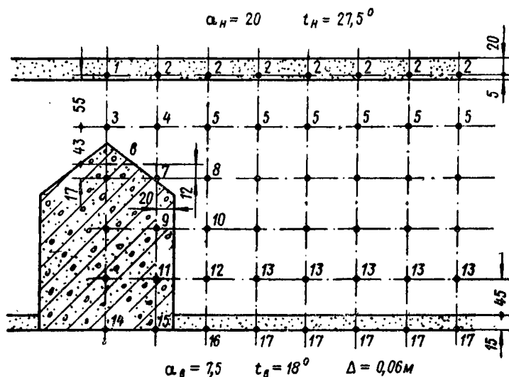
Рис. 58. Сетка температурного поля стыка панелей
