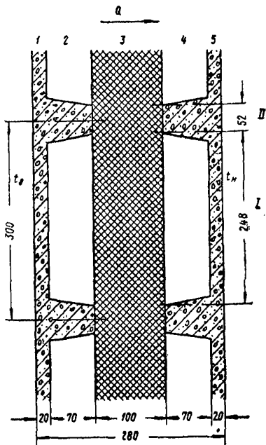
Рис. 50. К расчету сопротивления теплопередаче стеновой панели прокатной скорлупы
