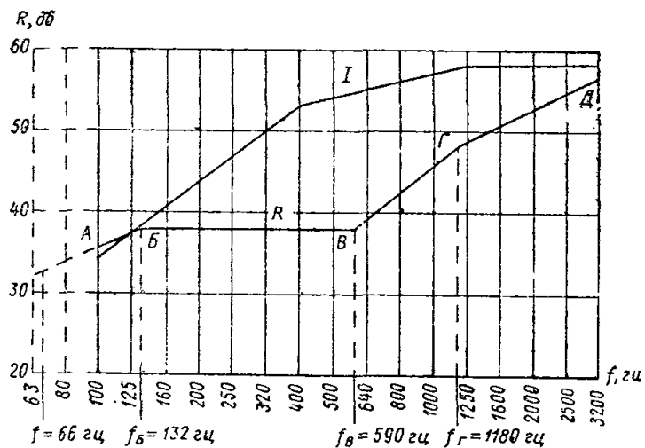
Рис. 97. Построение частотной характеристики звукоизолирующей способности железобетонной перегородки
