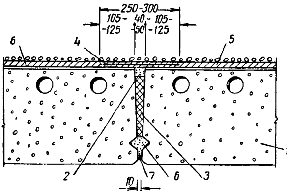
Рис. 28. Пример решения стыка панелей
