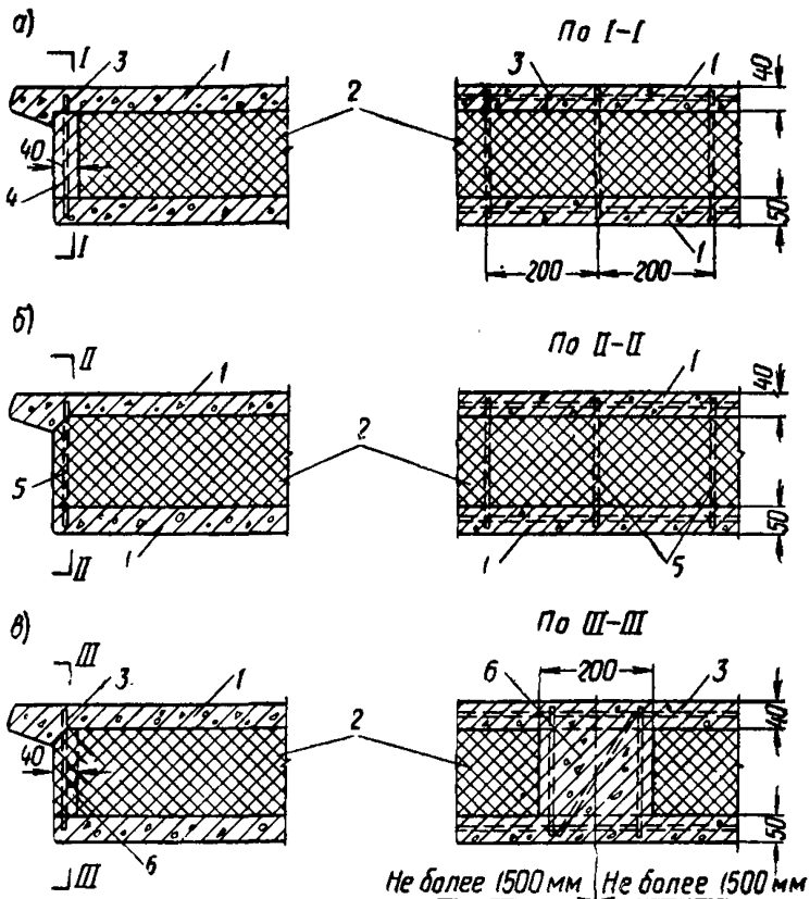
Рис. 3. Примеры соединительных связей в трехслойных панелях
