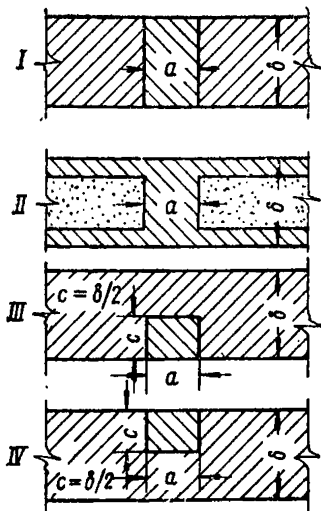
Рис. 55. Примеры теплопроводных включений в строительных конструкциях
