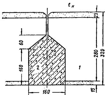
Рис. 56. Вертикальный стык керамзитобетонных панелей
