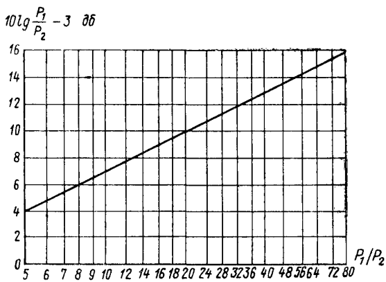
Рис. 89. График для определения величины 10 \lg \frac{P_1}{P_2} - 3 \text{ dB}
