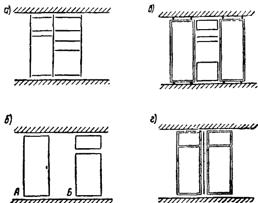
Рис. 17. Конструктивные схемы шкафов-перегородок
