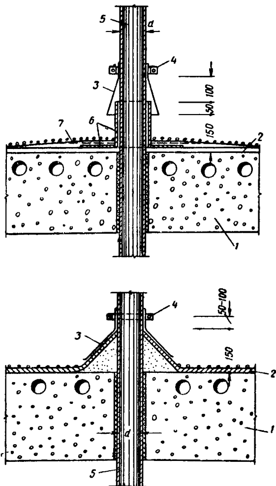
Рис. 31. Примыкание гидроизоляционного ковра к отдельно стоящим трубам
