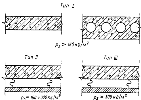
Рис. 85. Расчетные схемы перекрытий (без полов)
