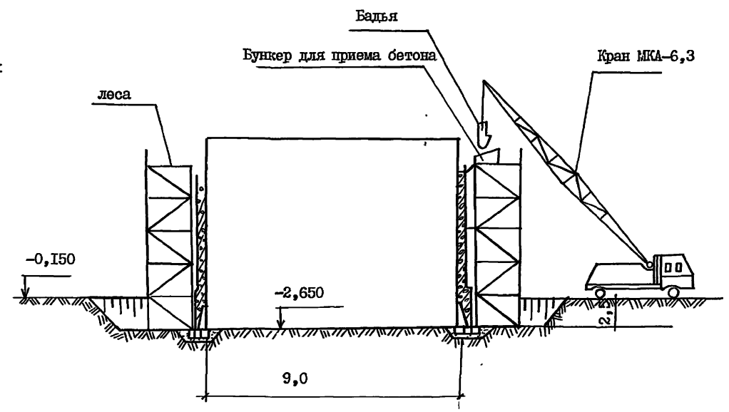
Схема погружения ошусного колодца в связных грунтах
