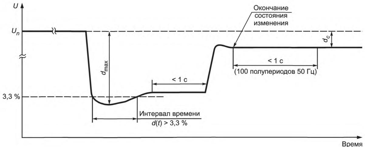
Рисунок В.2а — Пример для объяснения d -параметров
