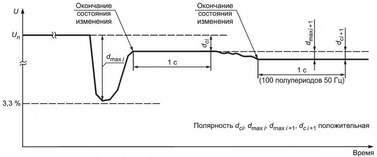
Рисунок В.2б — Пример для объяснения определений d -параметров при многократных условиях установившегося состояния
