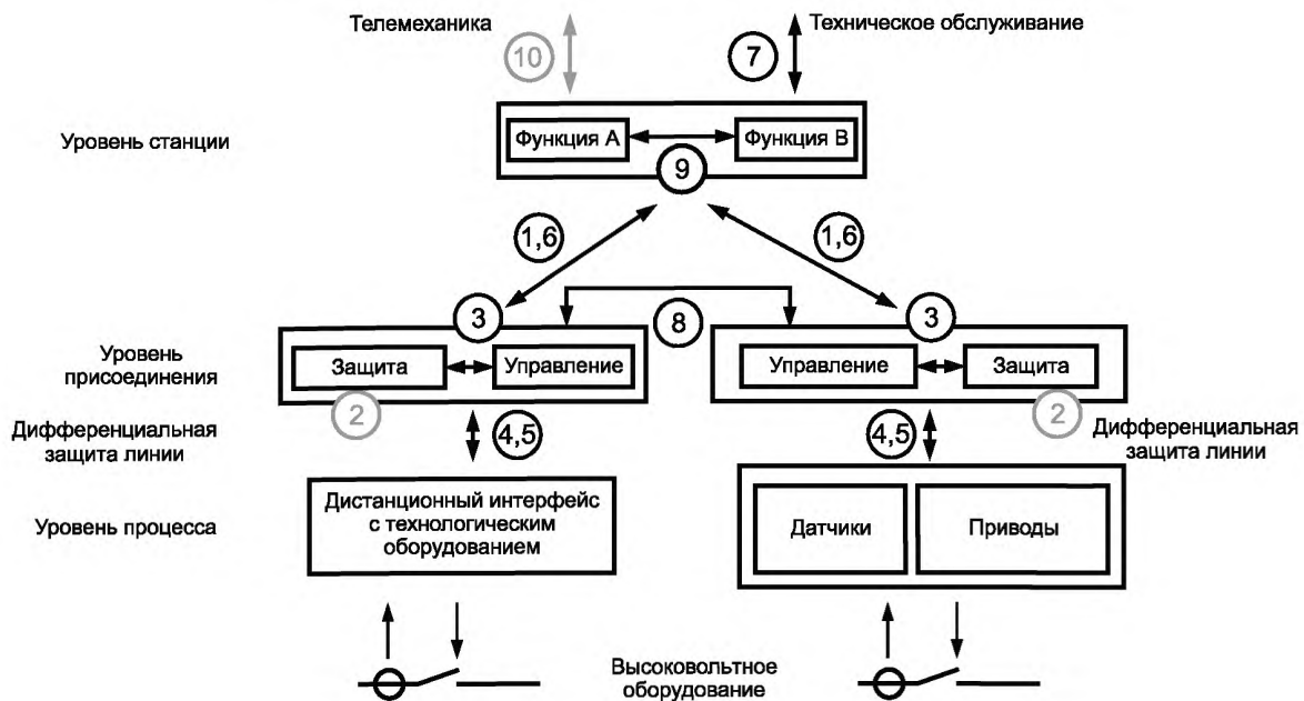
Рисунок ДА.1 — Модель интерфейсов системы автоматизации подстанции
