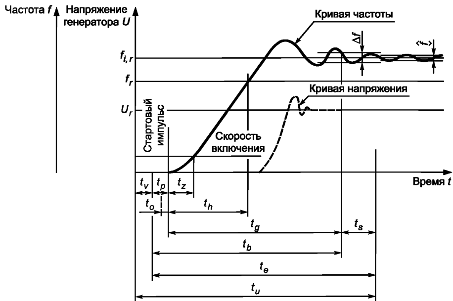
Рисунок 10 — Пусковые характеристики
