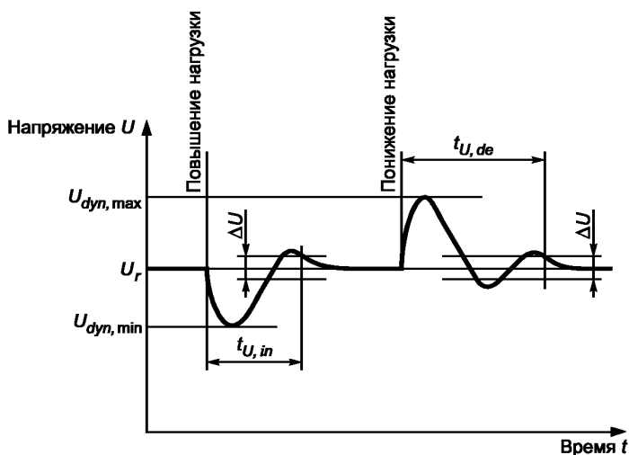
Рисунок 5 — Характеристики кратковременного напряжения без квадратурного статического отклонения напряжения компенсации
