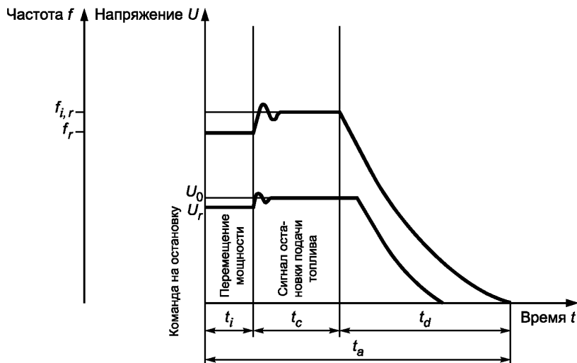
Рисунок 11 — Характеристики остановки
