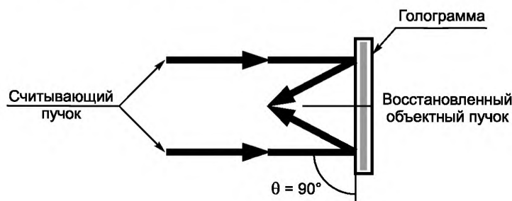
Осевая схема
