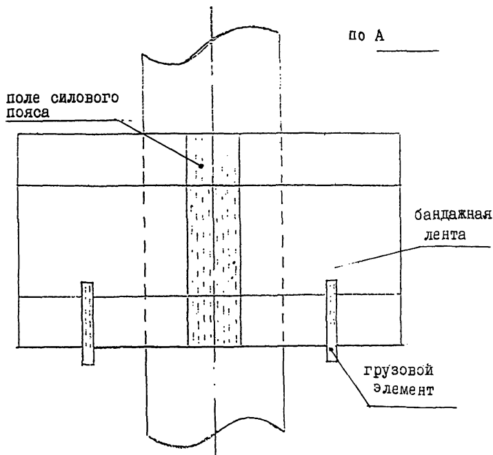
Рис. 4 Контейнер КТ-1400 на трубопроводе
