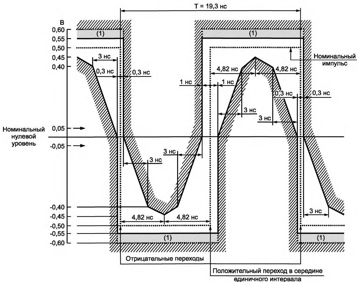
Рисунок Б.3 — Маска импульса 51840 кбит/с 1 (СМІ; «0»)
