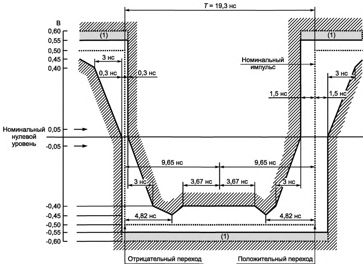
Рисунок Б.2 — Маска импульса 51840 кбит/с 1, 2 (СМІ; «1»)
