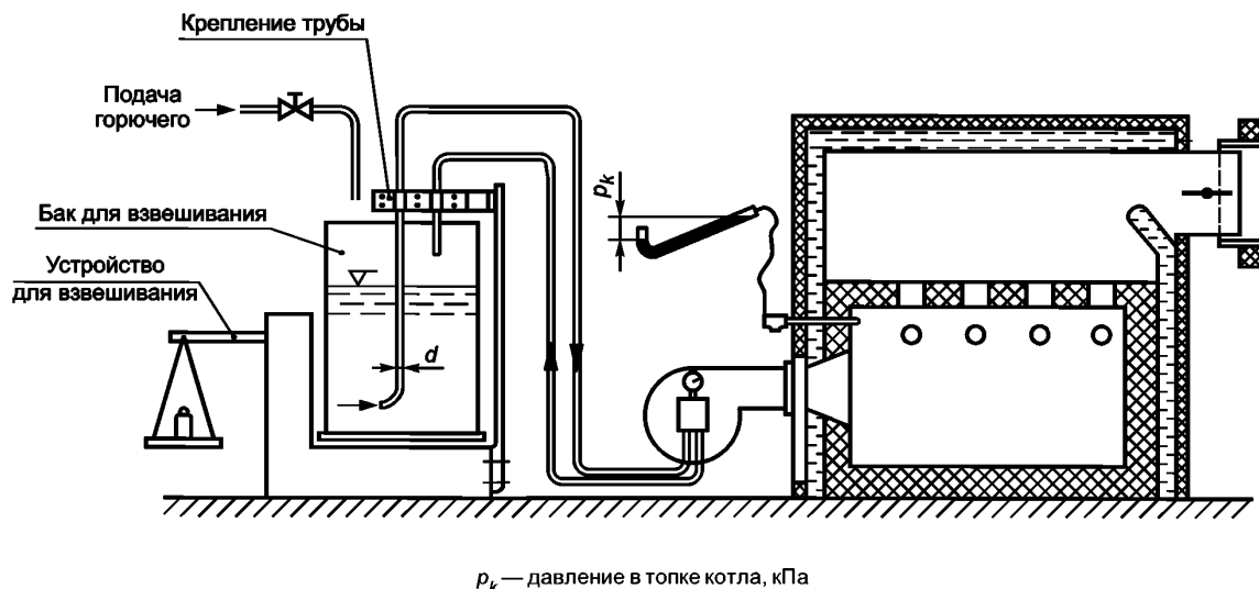
Рисунок 1 — Измерительная установка для определения расхода топлива
