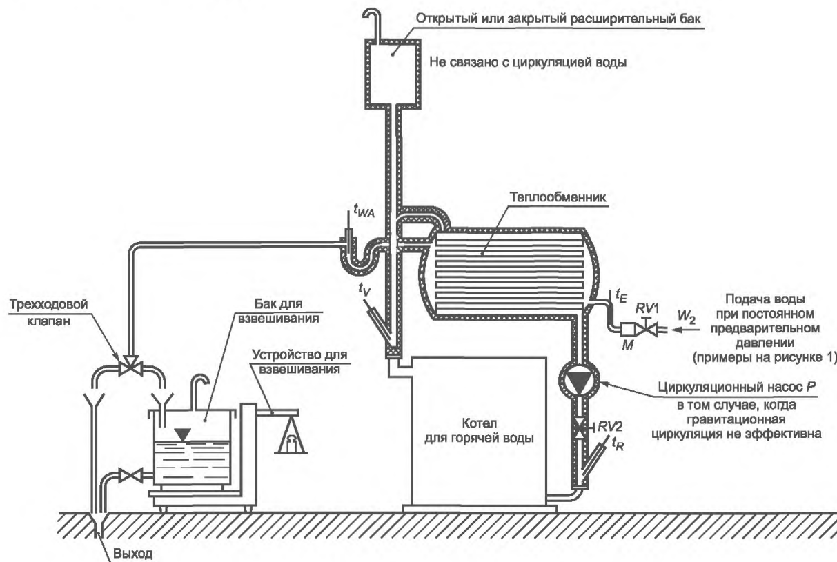
Рисунок А.1 — Испытательное оборудование с теплообменником
