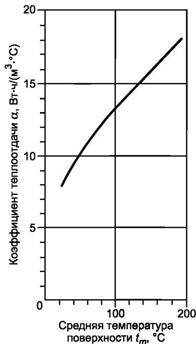
Рисунок А.4 — Значения полной теплоотдачи \alpha радиацией и конвекцией горизонтальным и вертикальным поверхностям при окружающей температуре t_L = 20 °С в зависимости от средней температуры поверхности t_m
