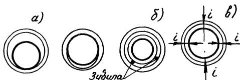
Рис. 4. Центровка труб со стороны гладкого конца / в раструбе уложенной трубы / а/ положение трубы в раструбе до центрирования; б/ подкладка зубил для центрирования; в) конечное положение трубы в раструбе при правильном центрировании i - величина кольцевого зазора
