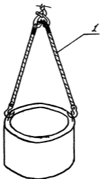
Рис. 8. Стрпоовка блоков котловца 1 - двухветвевой строп
