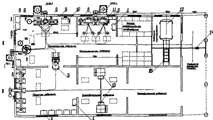
Рис.1. Примерная схема планировки и размещения оборудования цеха по изготовлению и антикоррозионной защите закладных деталей
