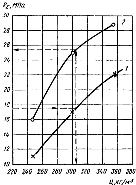
Рис. 2. Зависимость прочности бетона от фактического расхода цемента
