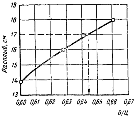
Рис. 1. Зависимость распыла раствора на встряхивающем столике от В/Ц
