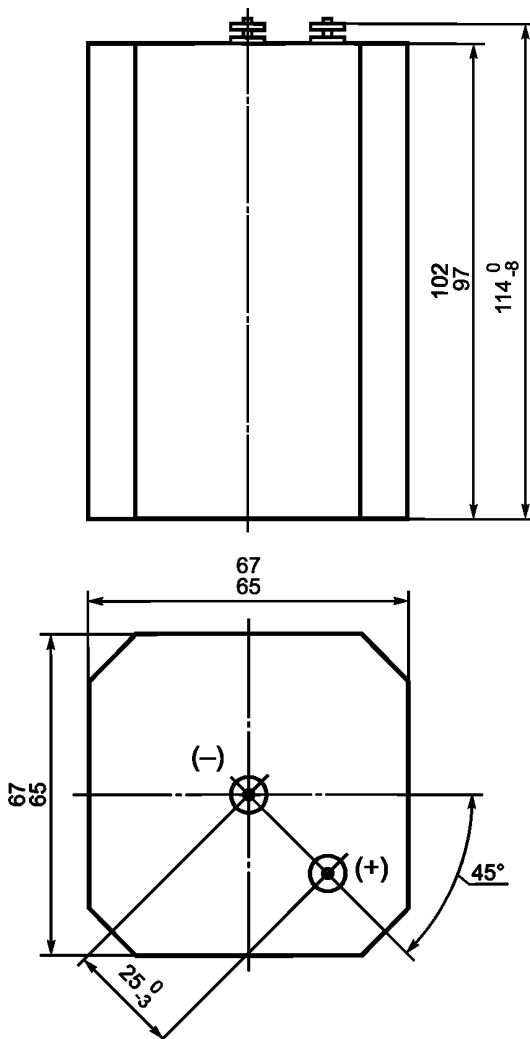
Рисунок 16 — Размеры батареи 4R25Y
