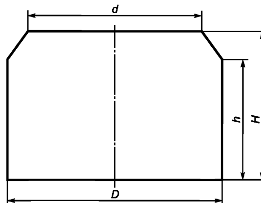
Рисунок 5 — Измерительный калибр для батарей категории 4
