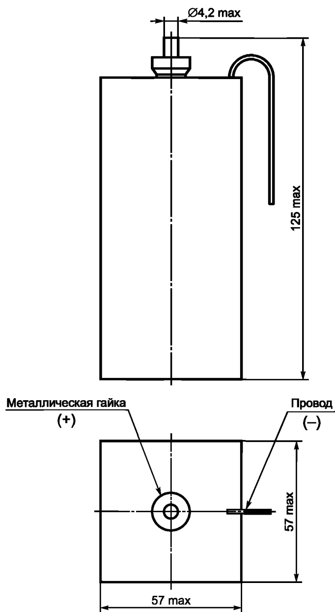
Рисунок 9 — Размеры батареи S4
