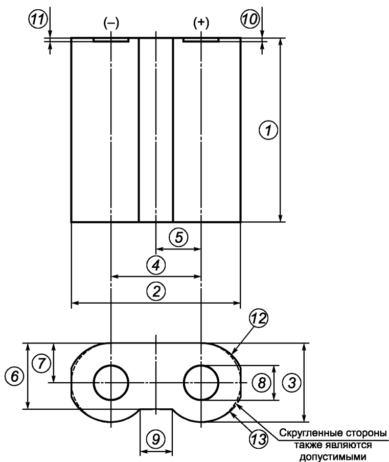
Рисунок 12 — Размеры батарей CR-P2, BR-P2
