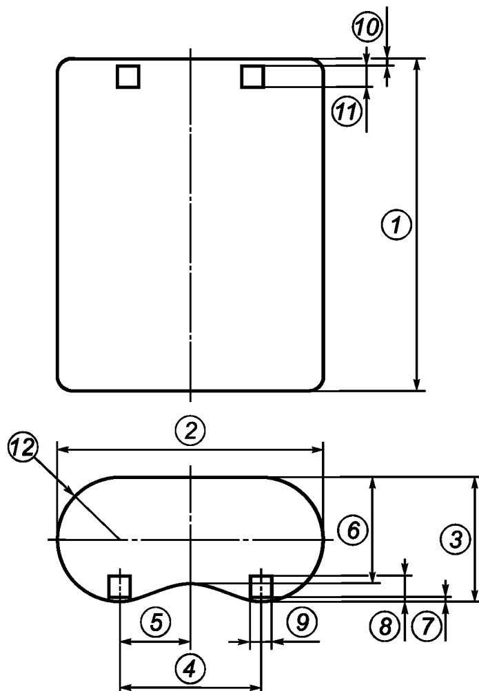
Рисунок 13 — Размеры батареи 2CR5
