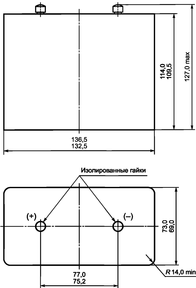
Рисунок 17 — Размеры батарей 4R25-2, 4LR25-2
