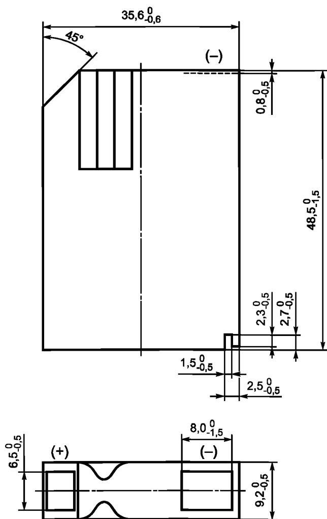
Рисунок 11 — Размеры батарей 4LR61
