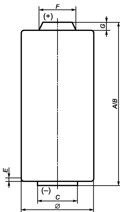
Рисунок 2 — Размеры батарей категории 2
