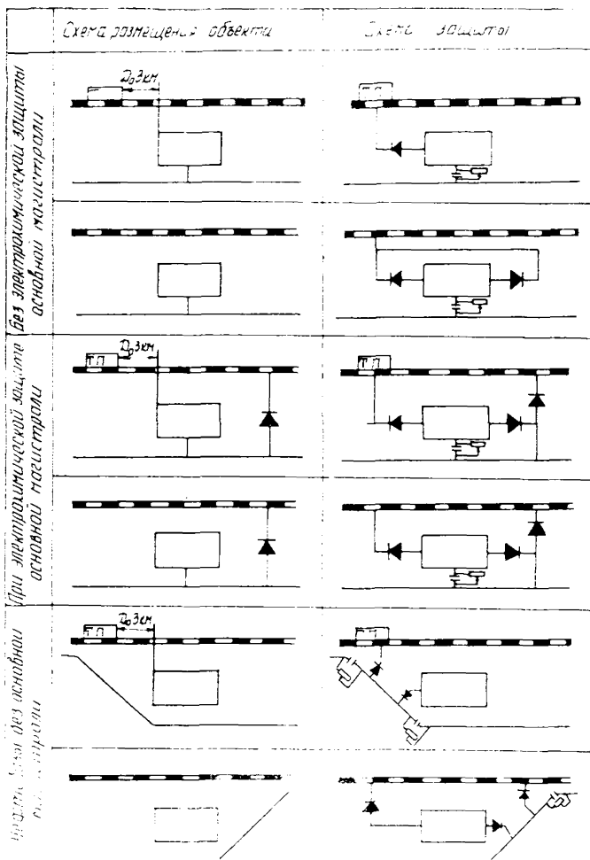
Рис. 5.3. Дренажная защита компрессорных и насосных станций и нефтебаз
