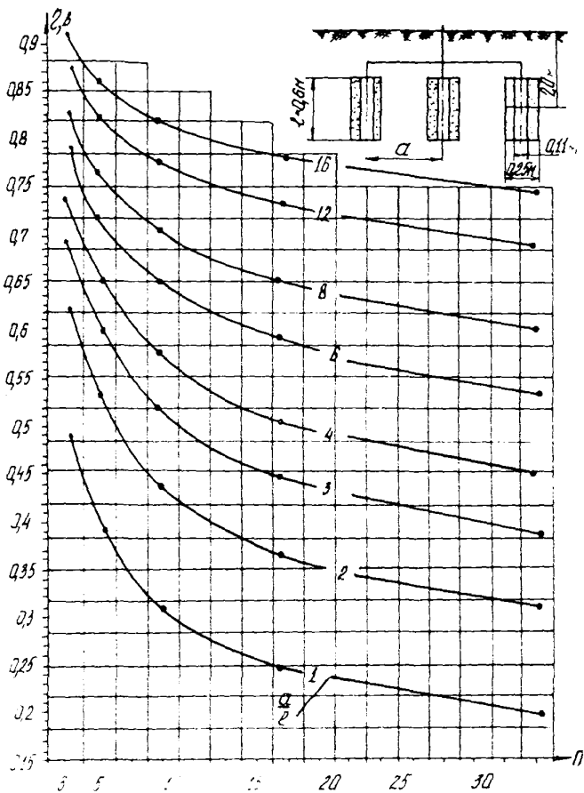
Рис. 1У.8. Зависимость коэффициента экранирования вертикальных упакованных протекторов Q_s от числа электродов n
