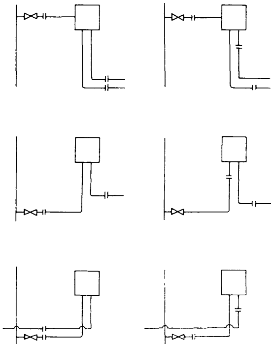
Рис.Ш.2. Основные схемы установки изолирующих фланцев на сосредоточенных объектах
