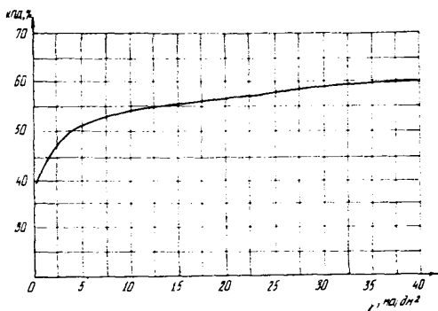
Рис. IV.7. Зависимость к.п.д. магниевого протектора от анодной плотности тока
