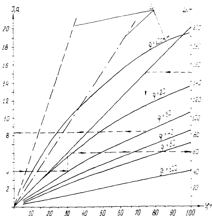
Рис.IV.3. Номограмма для определения защитного тока одиночного протяженного подземного сооружения на территории насосных и компрессорных станций и нефтебаз ( U_0 = 0,7 в; Z_B = 0,02 ом; R_{пер} (—) = 300 ом.м; R_{пер} (-.-.-) = 500 ом.м; R_{пер} (- - -) = 1000 ом.м)
