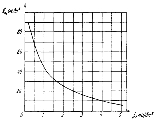
Рис.ИУ.6. Зависимость поляризационного сопротивления магневых протекторов от анодной плотности тока (упакованный протектор ППА-5 в глинистом грунте с удельным сопротивлением \rho_r = 25 \text{ ом}\cdot\text{м} )
