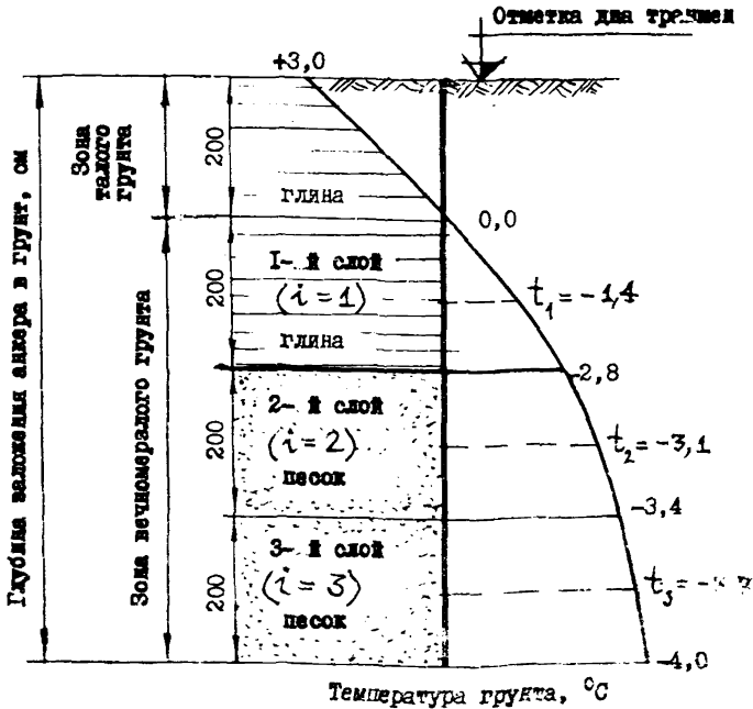
Рис.3. График распределения температур в грунте под трубопроводом.
