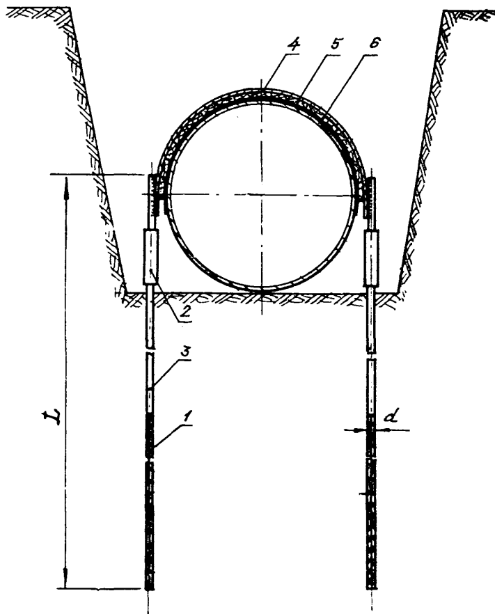
Рис.1. Стержневое анкеровое устройство
