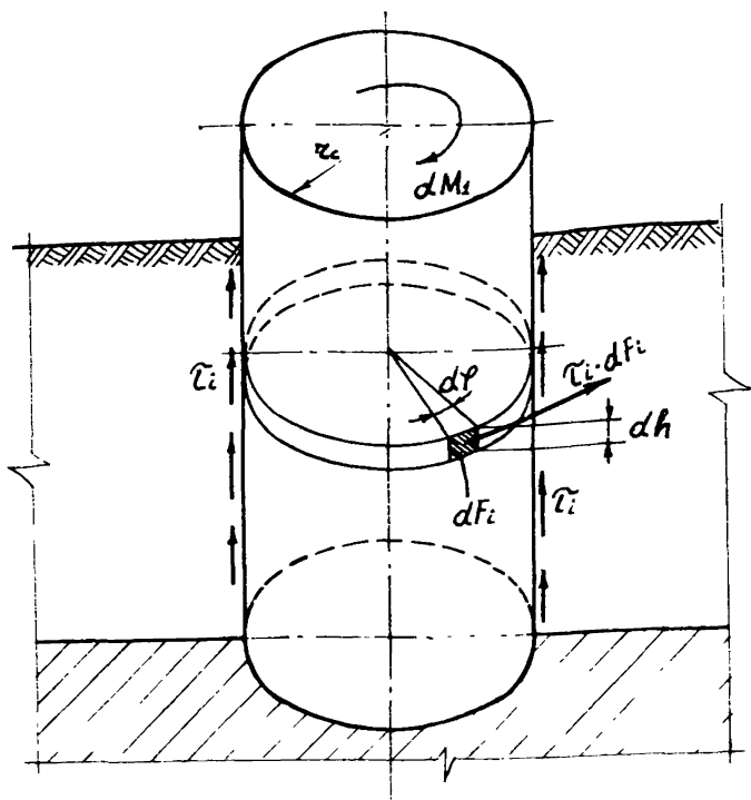
Рис.3. Расчетная схема для определения момента M_1
