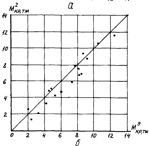
Рис. II. Диагональные графики распределения случайных отклонений для суглинка тугопластичного: а-подсчитанных по формуле (24); z_1' = 0,965 ; S_1' = 1,40 ; б- подсчитанных по формуле (21); z_1' = 0,970 ; S_1' = 0,91
