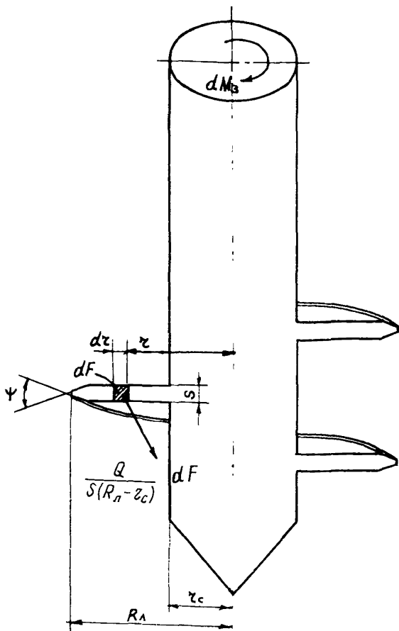
Рис.5. Расчетная схема для определения момента M_3
