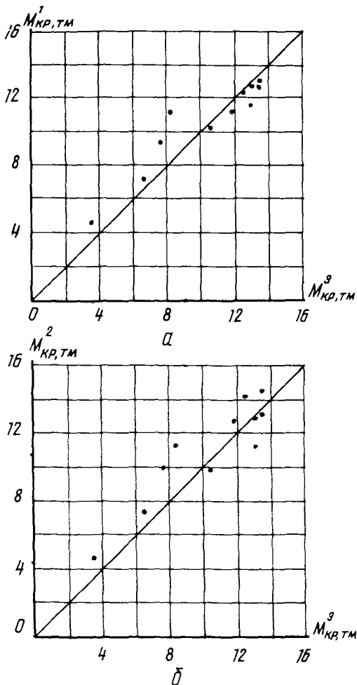
Рис.12. Диагональные графики распределения случайных отклонений для песка средней крупности и плотности: а-подсчитанных по формуле (24); z_7^1 = 0,935 ; S_7^1 = 1,25 ; б-подсчитанных по формуле (21); z_7^2 = 0,931 ; S_7^2 = 1,54
