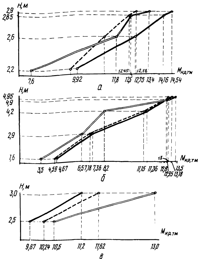
Рис. 10. Графики изменения величин крутящих моментов, вычисленных по формулам (24) (---), (21) (—) и определенных по приборам (===) для песков средней крупности и плотности: а—для свай с D_n=800 мм и d_c=330 мм; б—для свай с D_n=800 мм и d_c=219 мм; в—для свай с D_n=1000 мм и d_c=219 мм
