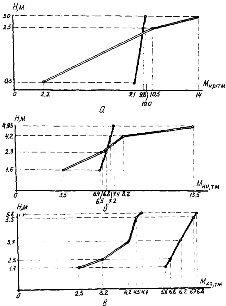
Рис. 8. Графики величин крутящих моментов M_{кр} , вычисленных по формуле (23) и определенных по приборам: а - для свай с D_n = 1000 мм, d_c = 219 мм, погруженной в плотный песок средней крупности; б - для свай с D_n = 800 мм, d_c = 219 мм, погруженной в песок средней крупности; в - для свай, погруженной в моренный суглинок: — — по тензометрическим приборам; — — по формуле (23)
