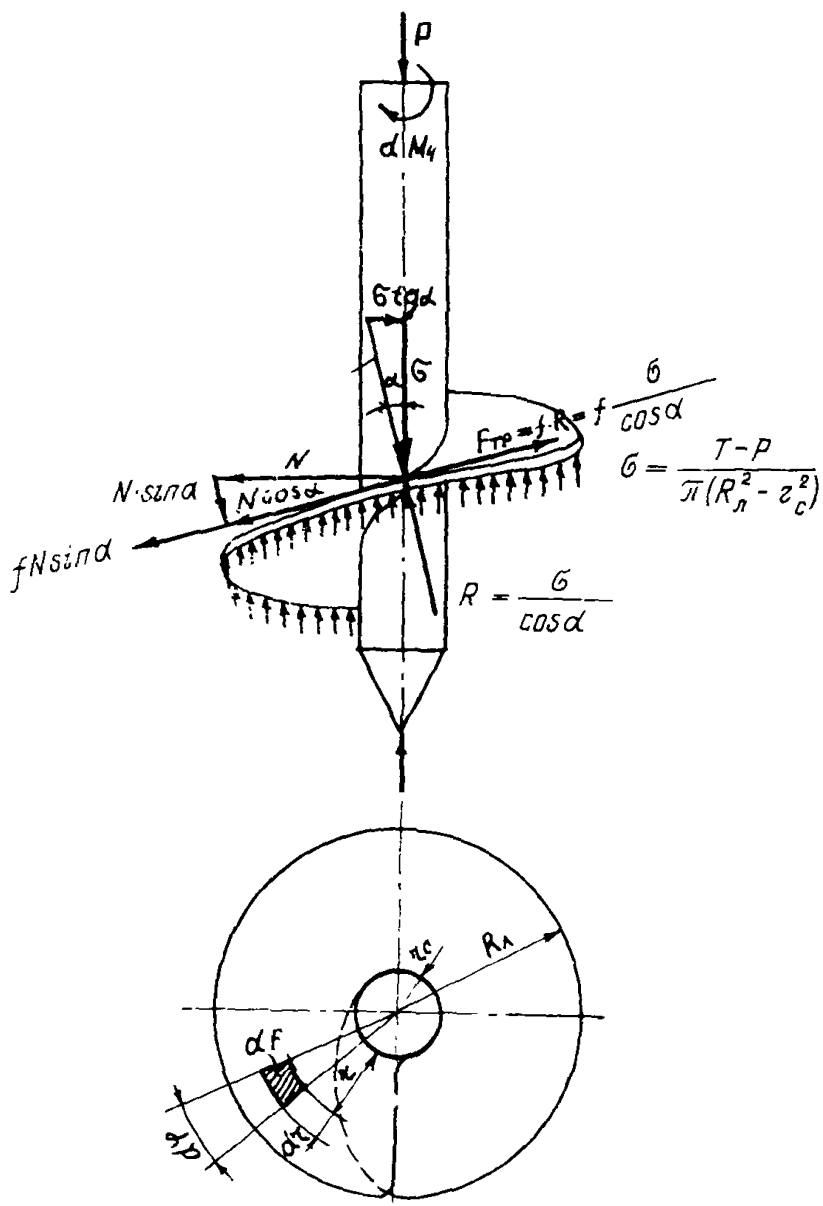
Рис. 3. Расчетная схема для определения момента M_4
