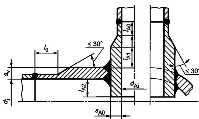
Рисунок А.2 — Усиление посредством сваренного патрубка с полным проплавлением
