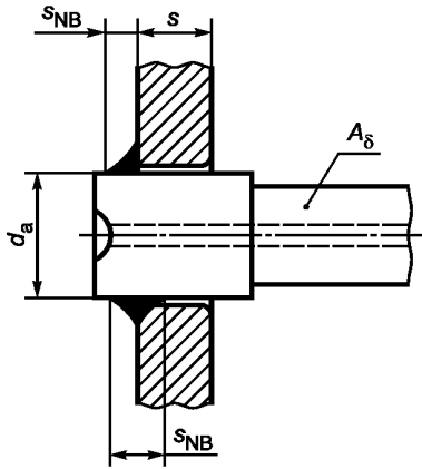
Рисунок D.12 — Приварной анкерный болт
