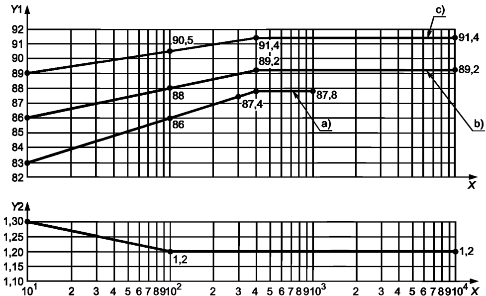
Y1 — КПД; Y2 — коэффициент избытка воздуха; X — тепловая мощность P_n , кВт a) \eta_k , отопительный котел, 30 % P_n ; b) \eta_k , отопительный котел, P_n ; c) \eta_k , низкотемпературный отопительный котел, P_n и 30 % P_n (только для котлов мощностью до 1000 кВт)
