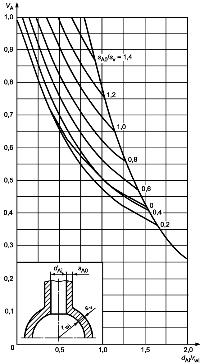
Рисунок В.15 — Значения коэффициента эффективности для сферических оболочек с вертикальным патрубком в зависимости от d_{Ai}/r_{wi} и s_{A0}/s_v при постоянном значении s_v/r_{wi}
