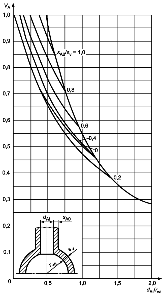
Рисунок В.16 — Значения коэффициента эффективности для сферических оболочек с вертикальным патрубком в зависимости от d_{Ai}/r_{wi} и s_{A0}/s_v при постоянном значении s_v/r_{wi}
