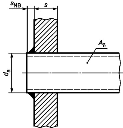
Рисунок D.13 — Приварная анкерная трубка
