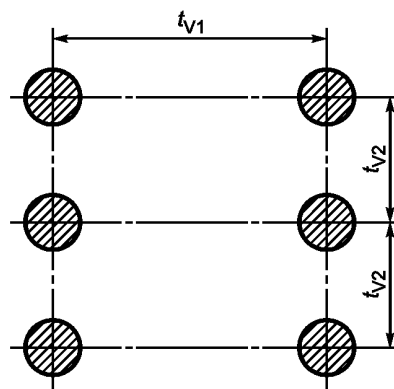
Рисунок D.9 — Равномерно расположенные анкерные крепления
