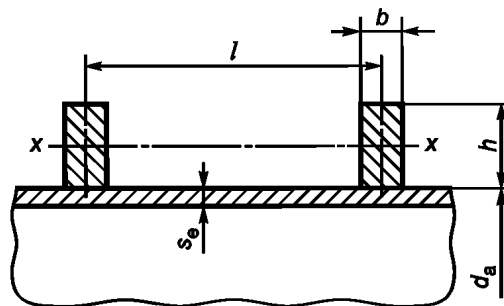
Рисунок Е.6 — Кольца жесткости
