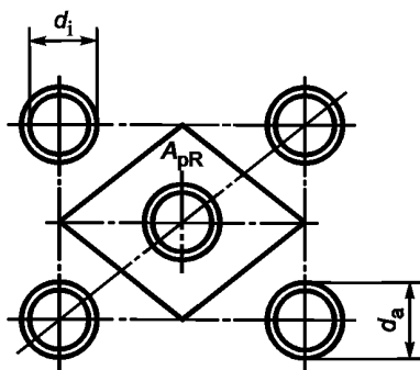
Рисунок D.15 — Площадь нагружения трубки — A_{pR}
