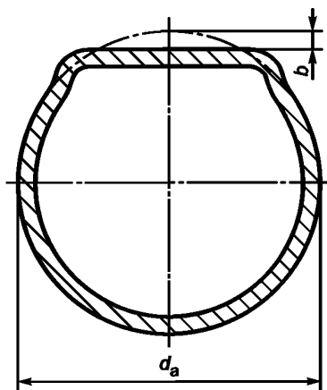
Рисунок Е.2 — Уплющение цилиндрических оболочек
