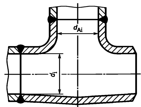
Рисунок А.5 — Патрубок, выполненный объемной штамповкой
