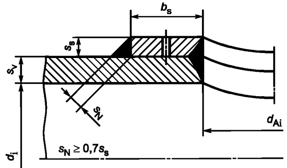
Рисунок А.7 — Отверстие с упрочняющим слоем (при температуре ≤ 250 °С)
