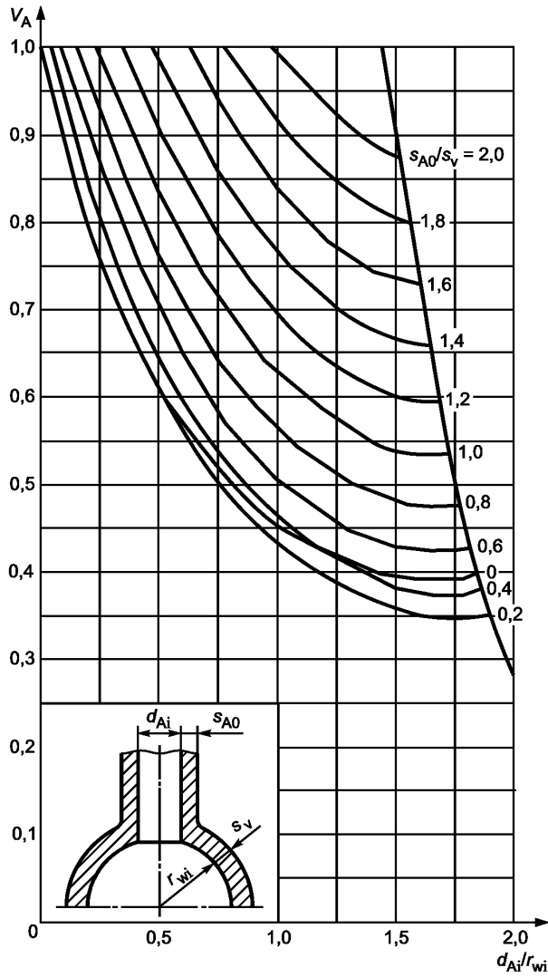
Рисунок В.14 — Значения коэффициента эффективности для сферических оболочек с вертикальным патрубком в зависимости от d_{Ai}/r_{wi} и s_{A0}/s_v при постоянном значении s_v/r_{wi}
