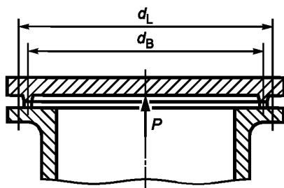
Рисунок D.3 — Свободно опертые и прикрепленные болтами плоские решетки
