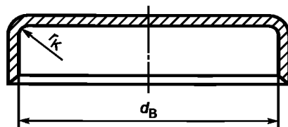
Рисунок D.2 — Круглое плоское днище с фланцем
