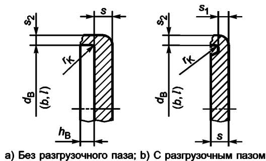
Рисунок D.1 — Сварные днища
