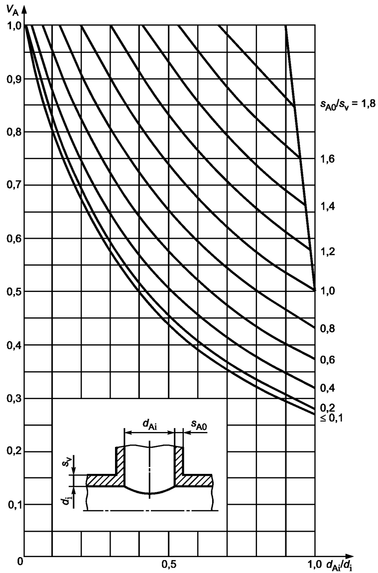
Рисунок А.21 — Значения коэффициента эффективности для цилиндрических оболочек с вертикальным патрубком, используемого для проверки правильности расчета готовых конструкций ( s_v/d_i = 0,05 )
