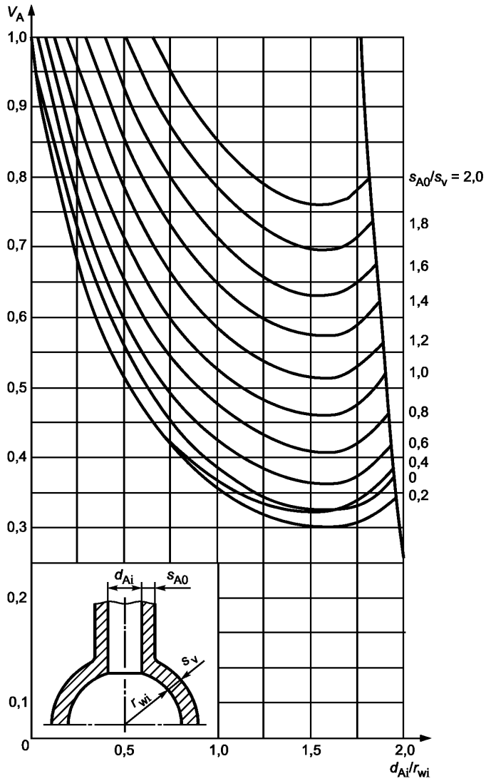
Рисунок В.13 — Значения коэффициента эффективности для сферических оболочек с вертикальным патрубком в зависимости от d_{Ai}/r_{wi} и s_{A0}/s_v при постоянном значении s_v/r_{wi}
