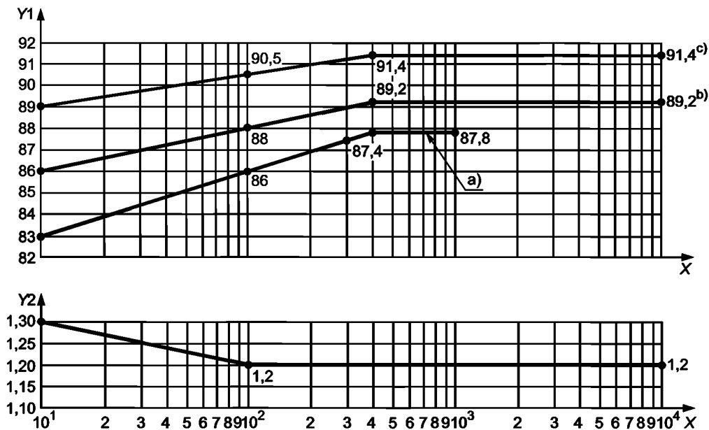
Y1 — КПД; Y2 — коэффициент избытка воздуха; X — тепловая мощность P_n , кВт; а) \eta_k , отопительный котел, 30 % P_n ; б) \eta_k , отопительный котел, P_n ; в) \eta_k , низкотемпературный отопительный котел, P_n и 30 % P_n (только для котлов мощностью до 1000 кВт).
