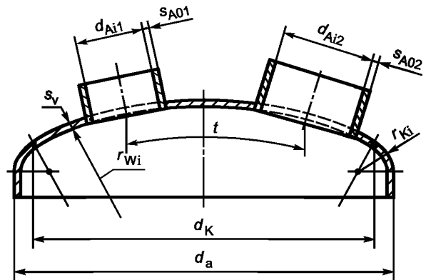
Рисунок В.2 — Выпуклое днище с отверстиями
