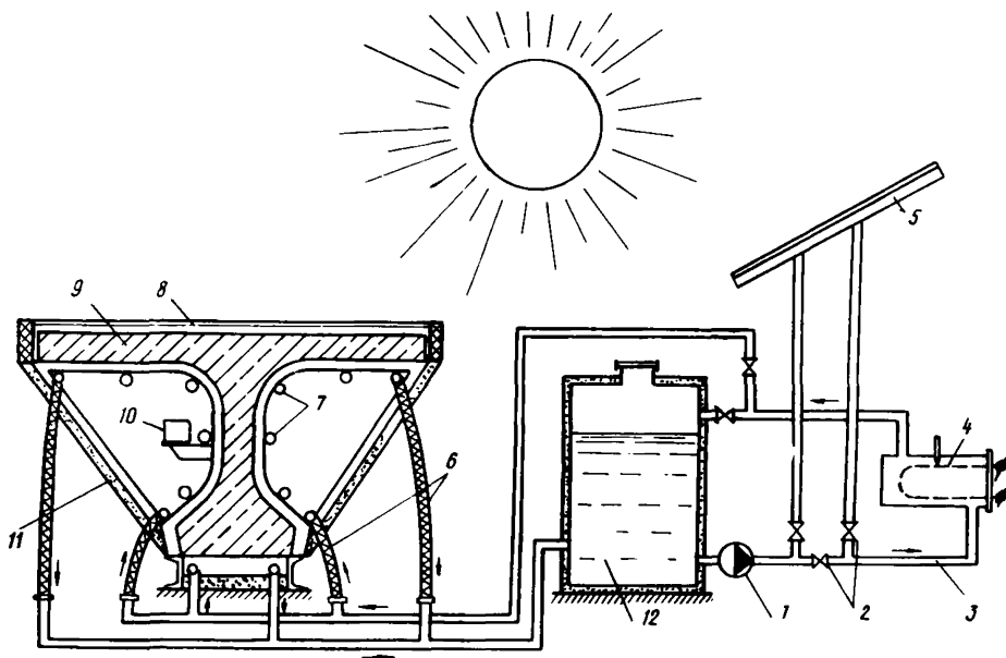
Рис.9. Принципиальная схема стенда для комбинированной гелиотермообработки балок пролетного строения моста с применением промежуточного теплоносителя
