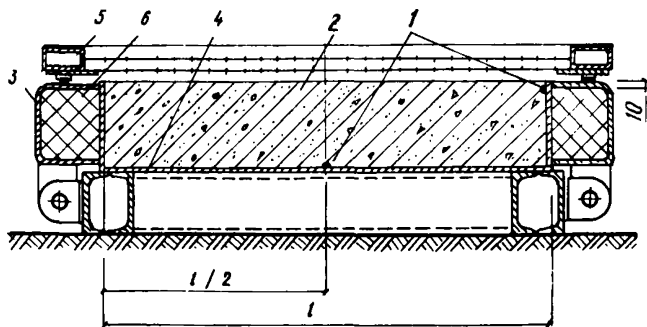
Рис.6. Схема установки контрольных термодатчиков в гелиотермоформе 1 - термодатчики; 2 - железобетонное изделие; 3 - борта гелиотермоформы; 4 - поддон гелиотермоформы; 5 - покрытие СВИАП; 6 - тепловая изоляция бортов гелиотермоформы
