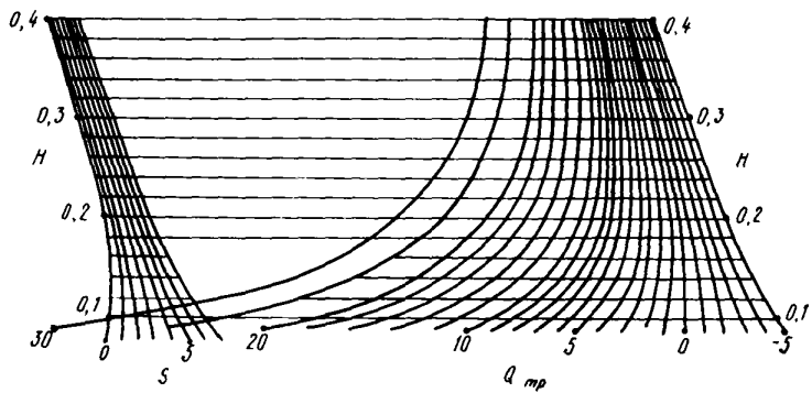
Рис.5. Номограмма для определения основных параметров КГТО изделий (суточная прочность бетона 70 % R_{28} )
