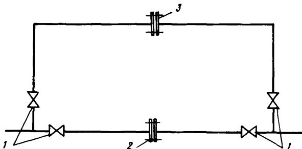
Рис.7. Принципиальная схема основного и байпасного паропровода с установленными на них расходными диафрагмами
