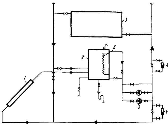
Рис.8. Принципиальная схема системы промышленного геотеплоснабжения для геотермообработки железобетонных изделий
