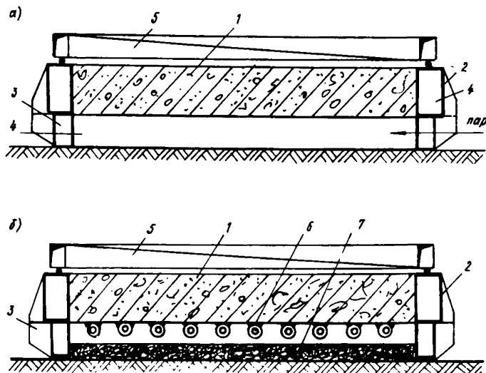
Рис.1. Принципиальные схемы гелиотермоформ для комбинированной гелиотермообработки железобетонных изделий при стендовом способе производства
